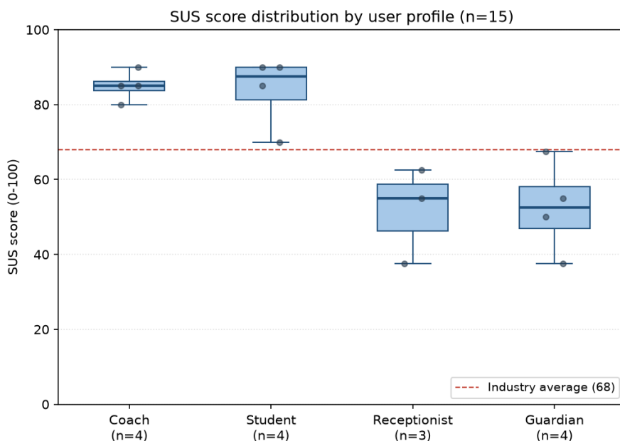
Figura 7: Distribución de puntuaciones SUS por perfil (diagrama de caja), generado por scripts/sus-boxplot.py a partir de docs/mediciones/sus/respuestas.csv . La línea punteada marca la media de la industria (SUS = 68).
