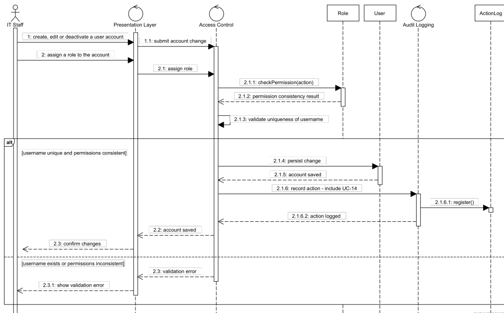
Figura 29: Diagrama de secuencia — CU-11 Gestionar usuarios, roles y permisos
