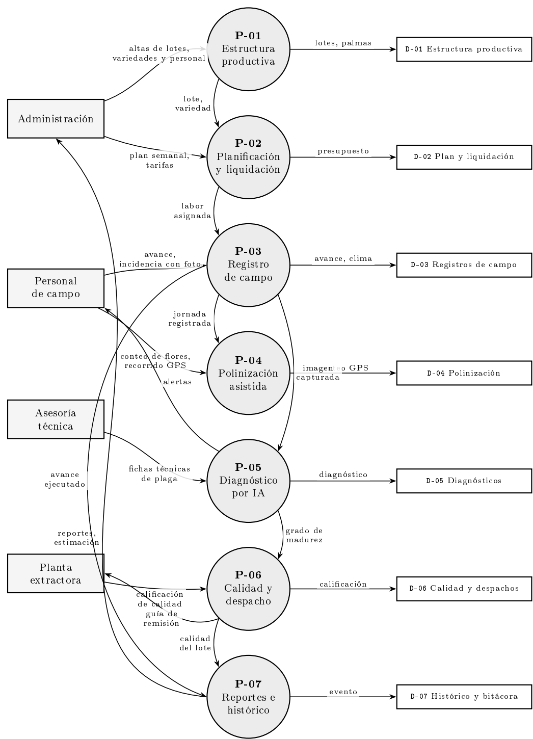
Figura 15: DFD de nivel 1 — descomposición del SIMPA en siete procesos.
