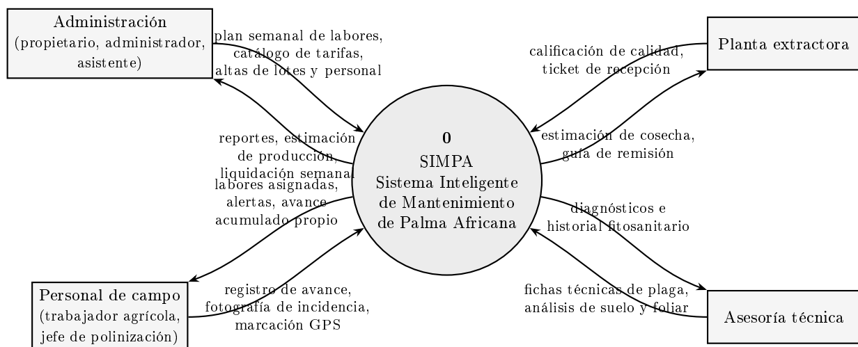
Figura 14: DFD de nivel 0 — diagrama de contexto del SIMPA.
