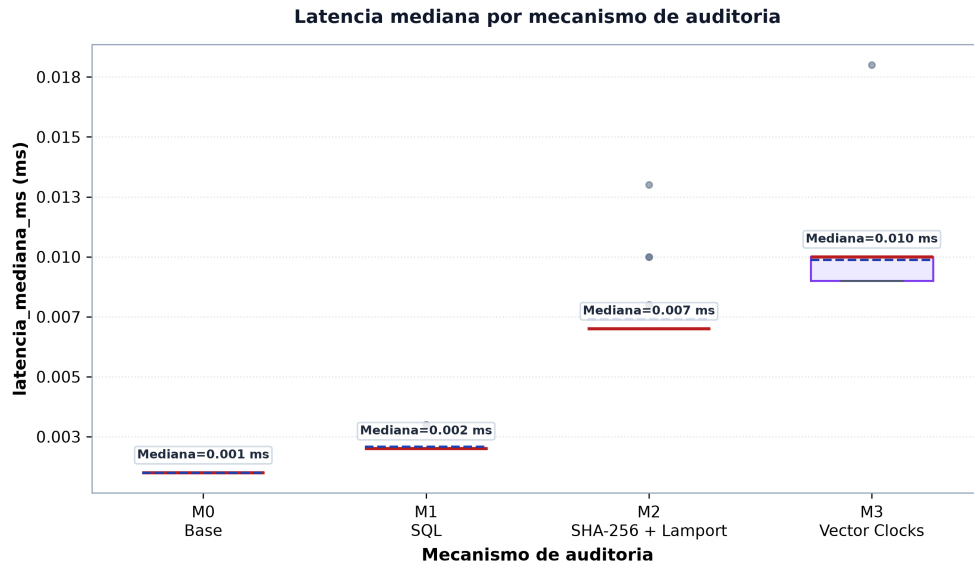
Figura 9: Distribución de las 40 observaciones de latencia_mediana_ms por mecanismo, expresadas en milisegundos y obtenidas de exp1_concurrencia.csv .
