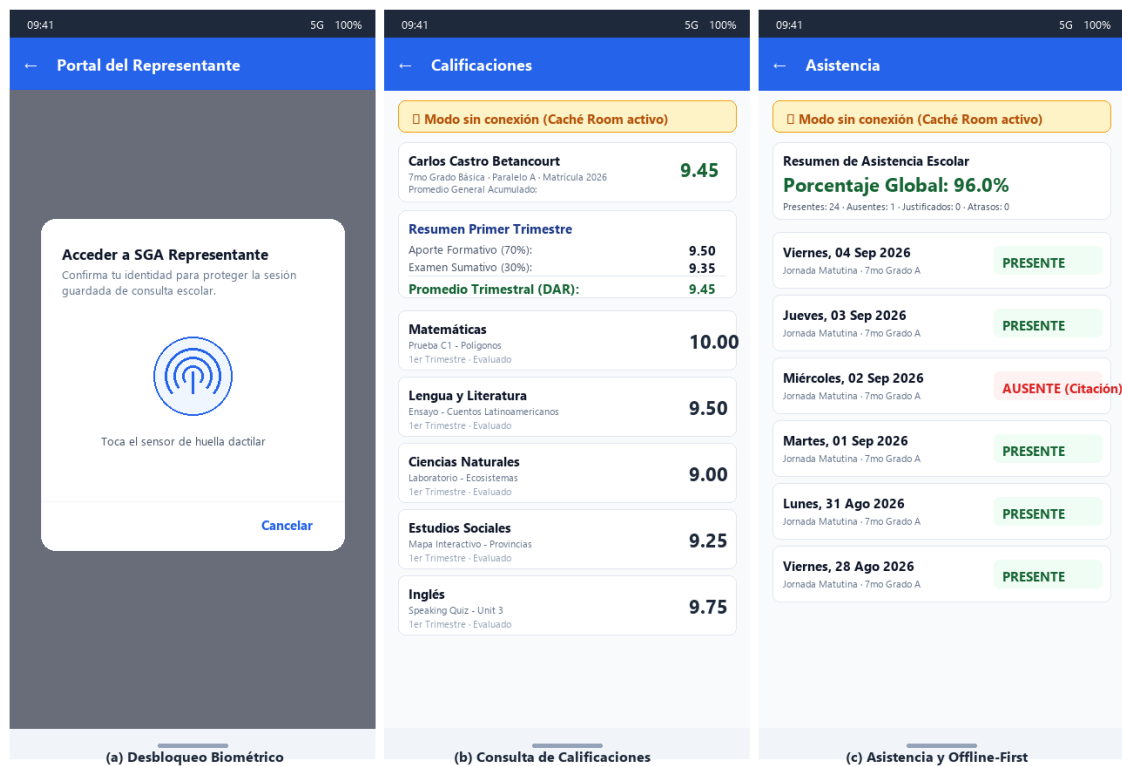
Figura 6: Interfaz de la Aplicación Móvil para Representantes (Kotlin + Jetpack Compose): (a) Desbloqueo seguro de sesión mediante autenticación biométrica nativa ( BiometricPrompt ), (b) Consulta académica con soporte de caché desconectado offline-first en SQLite Room, y (c) Módulo de asistencia y resumen escolar con reconciliación automática mediante WorkManager .
