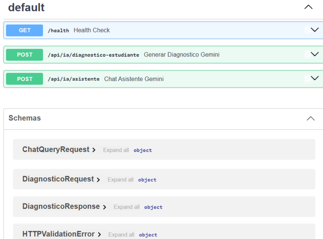
Figura 8: Documentación de la API del microservicio de IA con las rutas de salud, diagnóstico de estudiante y asistente visibles.
