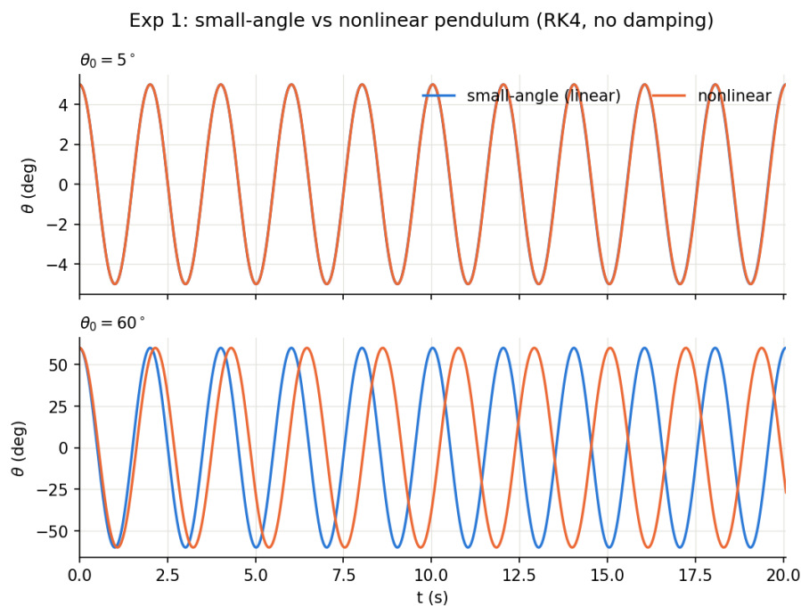
圖 1: 實驗一： \theta(t) 。上： \theta_0 = 5^\circ 兩條曲線幾乎重合；下： \theta_0 = 60^\circ 非線性解逐漸落後。
