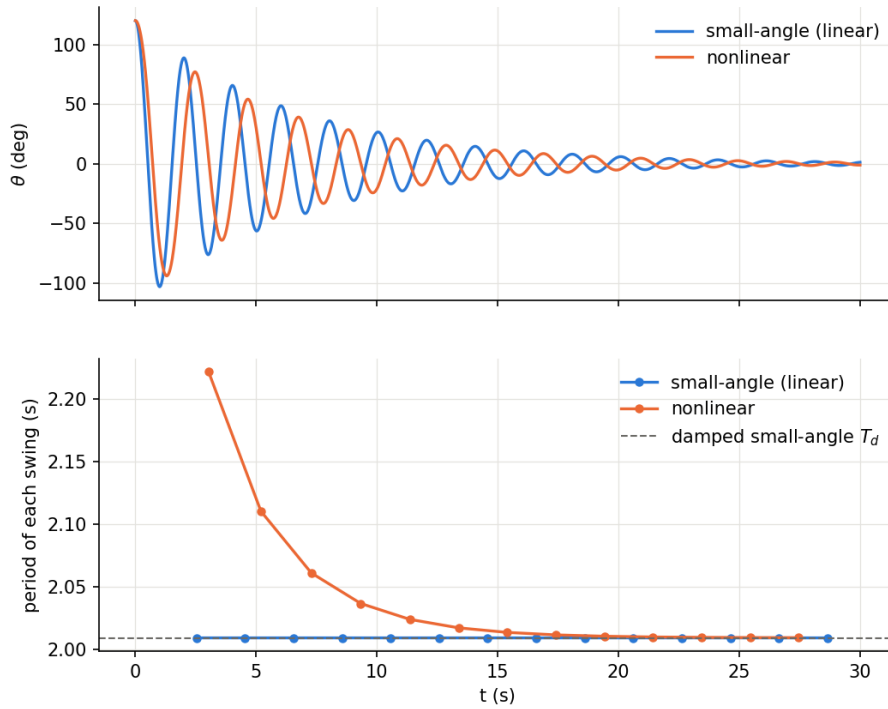
圖 6: 實驗四：上為 \theta(t) ；下為每次擺動的週期，虛線為 T_d 。
