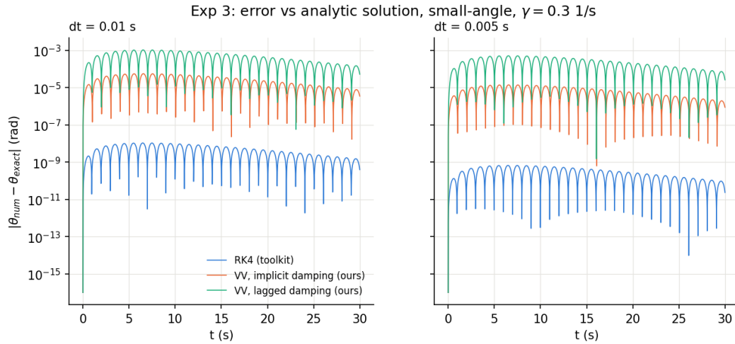
圖 4: 實驗三： |\theta_{\text{num}} - \theta_{\text{exact}}| 隨時間變化（對數座標）。
