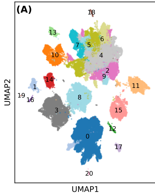
Leiden clusters
