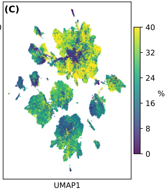
Ribosomal RNA (%)
