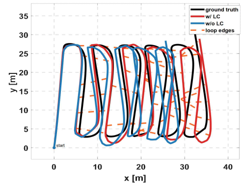
그림7. Loop closure 적용 여부에 따른 SLAM 경로 비교
