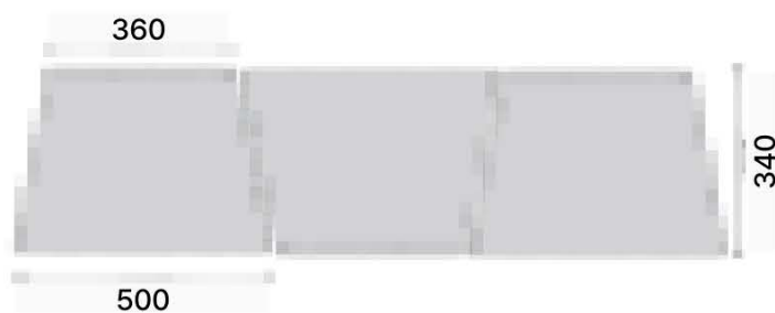
· 마감(캡) 블록 조립도
