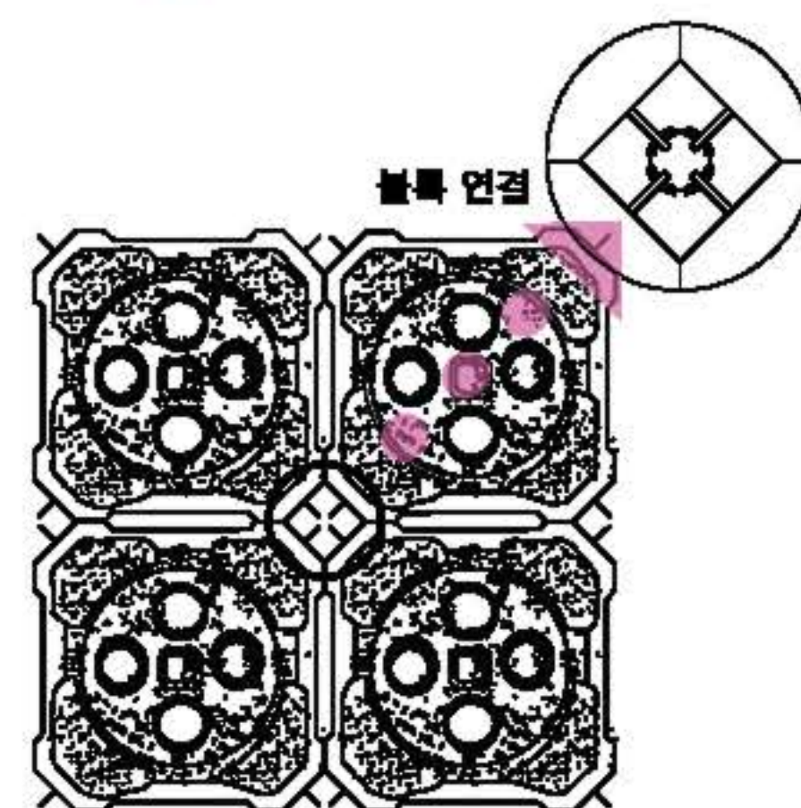
시공평면도
