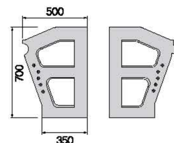
반블록 평면도
