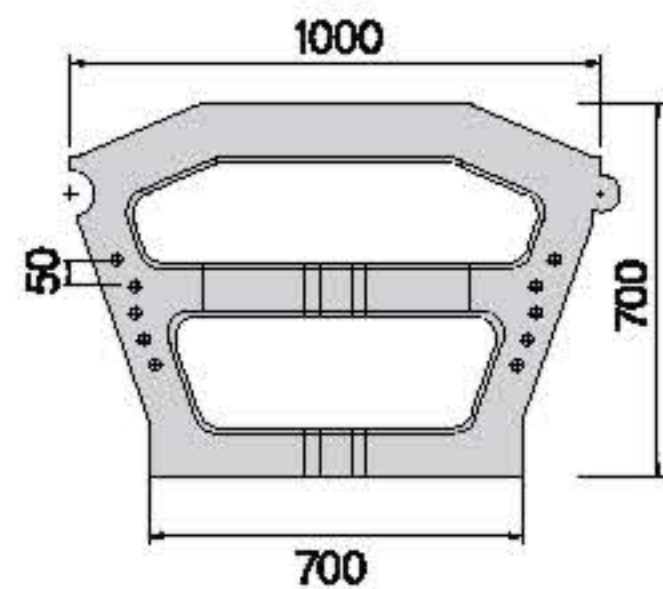
평면도
