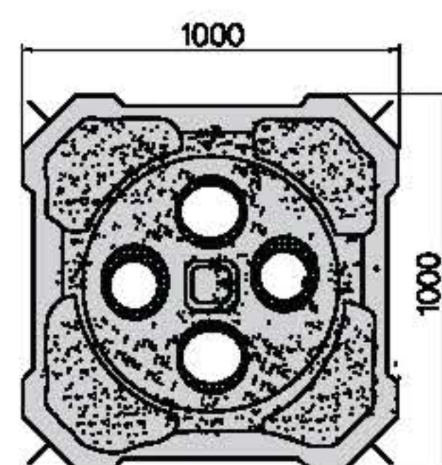
평면도
