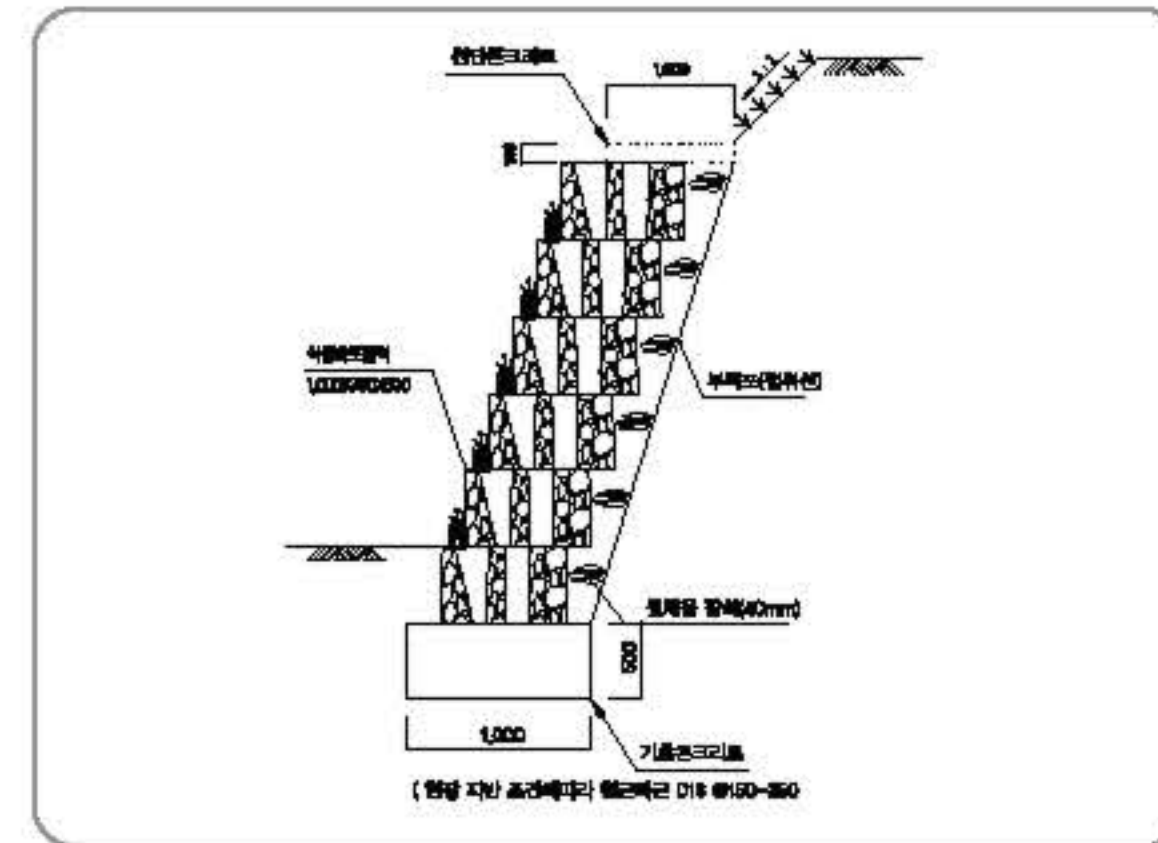
시공단면도
