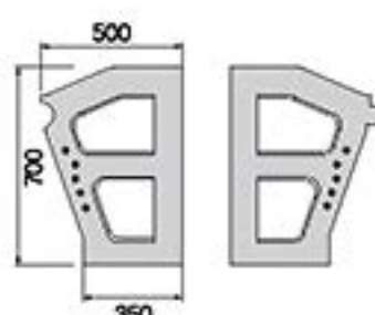
○ 반블록 평면도
