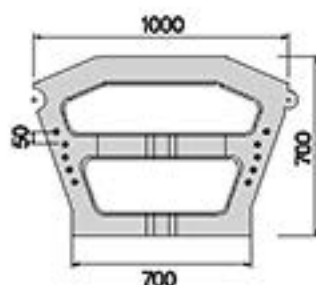
○ 평면도
