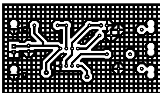
figure 4 : typon de la couche BOTTOM à l'échelle 1, sans miroir
