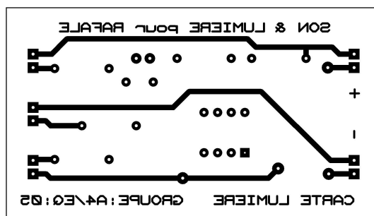
figure 3 : typon de la couche TOP à l'échelle 1, avec miroir
