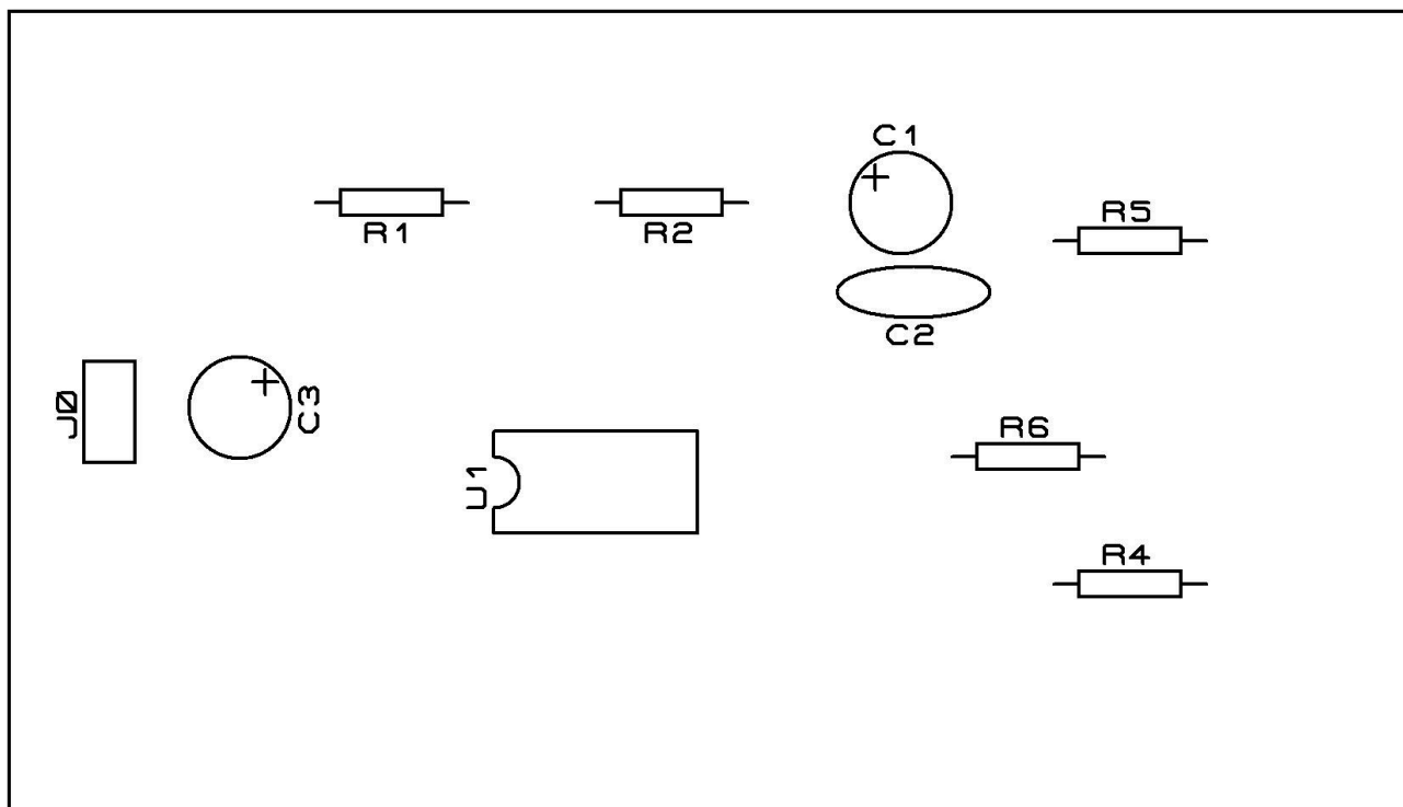
figure 6 : Schéma d'implantation du dessus
