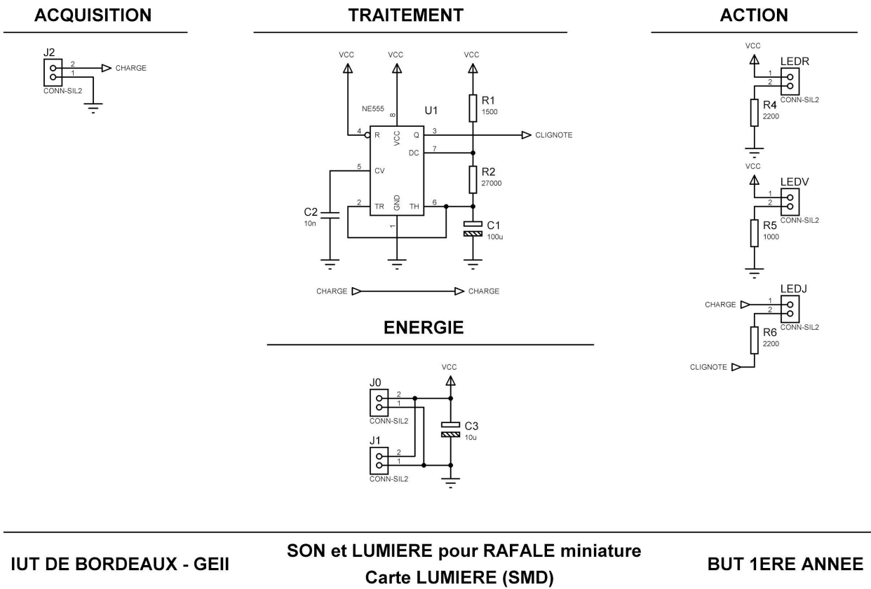
figure 1 : schéma électrique de la « carte lumière » du « système sonore et lumineux »
