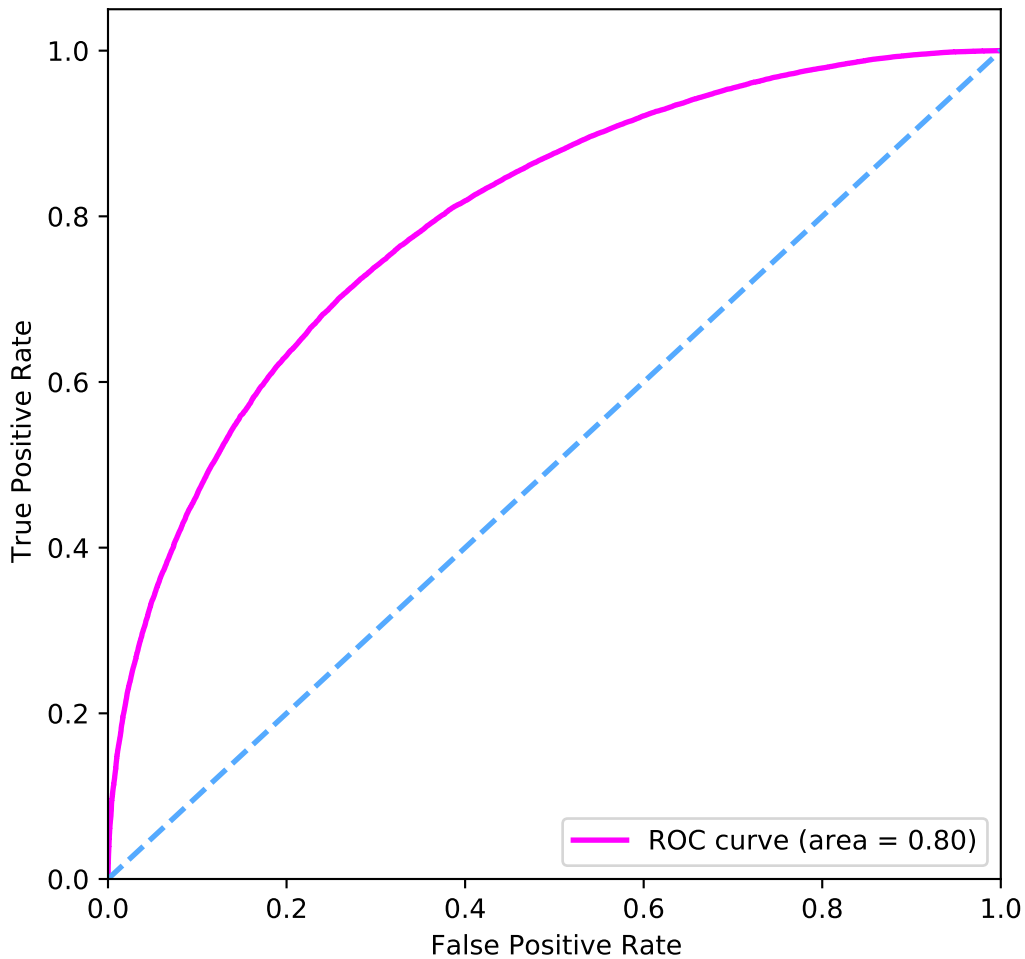
ROC catboost
