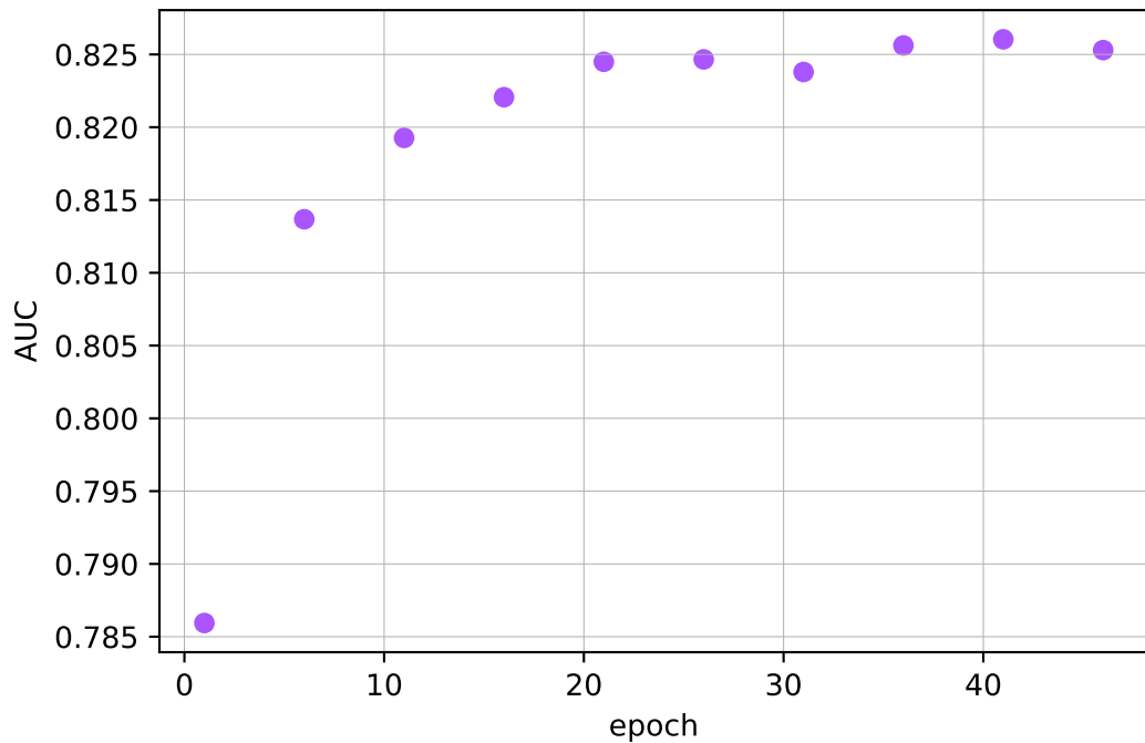
AUC v odvisnosti od epoch
