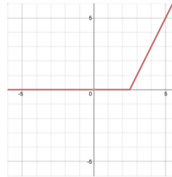
(c) \begin{cases} 2x - 5 & x \geq 2.5 \\ 0 & x < 2.5 \end{cases}
