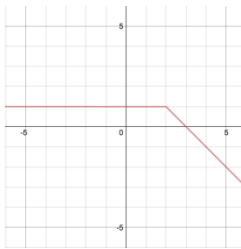
(e) \begin{cases} -x + 3 & x \geq 2 \\ 1 & x < 2 \end{cases}
