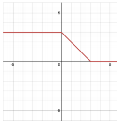
(f) \begin{cases} 3 & x \leq 0 \\ 3 - x & 0 < x \leq 3 \\ 0 & x > 3 \end{cases}
