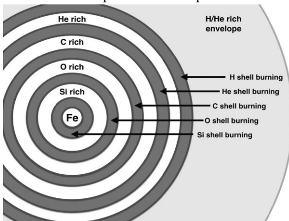
Рисунок 10.4 «Лукообразная» структура звезды с массой более 800 \text{ мкг/м}^3 состоит из различных элементов, подвергающихся «сжиганию оболочек», которые затем сливаются, образуя следующий слой М. Элементы располагаются в последовательности H, He, C, O, Si, Fe (другие элементы встречаются в относительно небольших количествах). Железо не может быть успешно синтезировано, поскольку реакция синтеза становится эндотермической.
