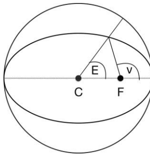
Рисунок 4.2 Эксцентриситет и истинная аномалия кеплеровской орбиты. Тела вращаются по эллипсам вокруг фокуса (F). Эксцентрисическая аномалия описывает угол, который вращающееся тело образовывало бы с центром эллипса (C), если бы оно двигалось по круговой орбите. Следовательно, эксцентрисическая и истинная аномалия эквивалентны, когда орбита круговая.
