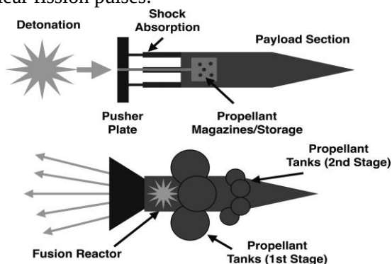
Рисунок 19.3 Внешняя и внутренняя ядерные двигательные установки (верхняя и нижняя). Эти упрощенные схемы иллюстрируют конструкции кораблей «Орион» и «Дедал» соответственно.
