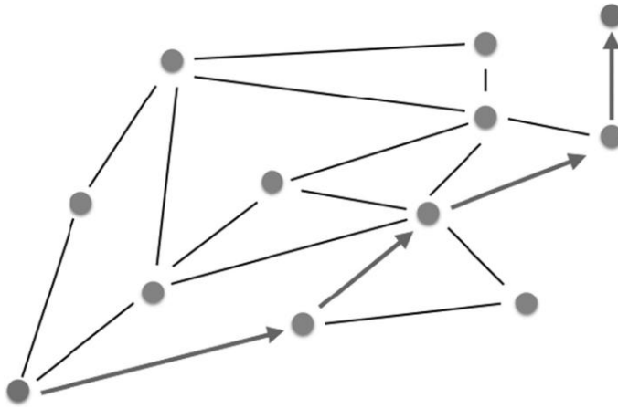
Рисунок 15.1 Алгоритм A* в действии. Чтобы найти кратчайший путь между самой левой и самой правой вершинами этого графа (обозначены стрелками), алгоритм вычисляет функцию стоимости для всех возможных вершин, чтобы перейти к следующей вершине, используя расстояние между этой вершиной и пунктом назначения в качестве эвристики (уравнение 15.3).
