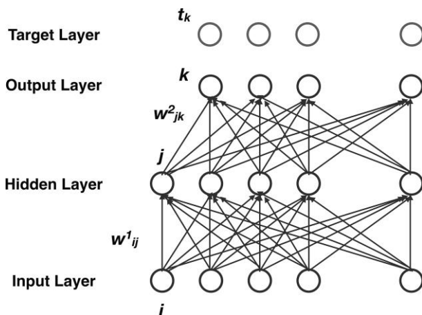
Рисунок 15.2 Трехслойная нейронная сеть обратного распространения ошибки. Каждый нейрон i во входном слое соединен со скрытым слоем с помощью веса соединения w^1_{ij} . Затем каждый нейрон в скрытом слое соединен с нейроном в выходном слое k с помощью веса w^2_{jk} . Выходы x_k сравниваются с целевыми выходами t_k .
