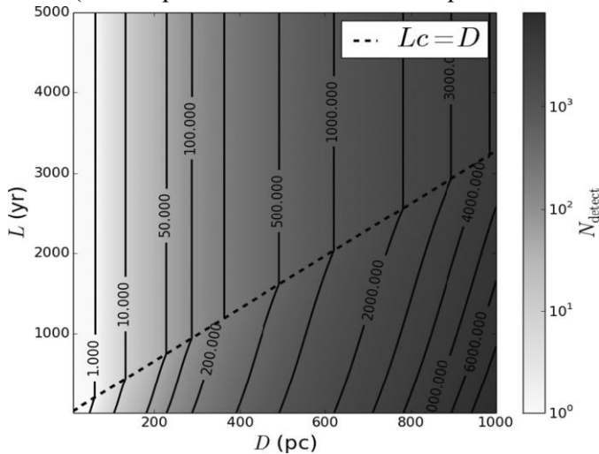
Рисунок 27.2 Количество обнаруживаемых цивилизаций как функция времени жизни трансляции цивилизации L и дальности трансляции D (см. уравнение (27.6)). Заметим, что для долгоживущих сигналов обнаруживаемость зависит только от дальности. Как только Lc \leq D (пунктирная линия), обнаруживаемость зависит от ширины сферической оболочки, создаваемой изотропным сигналом.
