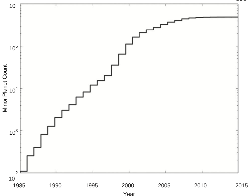
Рисунок 25.2 Общее количество зарегистрированных малых планет (астероидов, комет и карликовых планет) в зависимости от времени. За последние несколько десятилетий было обнаружено чрезвычайно большое количество таких объектов. Данные предоставлены Центром малых планет Международного астрономического союза.
