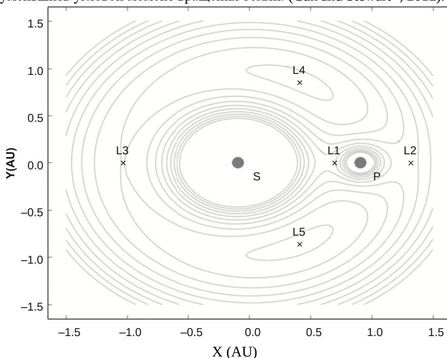
Рисунок 4.15 Точки Лагранжа системы звезда-планета (в системе отсчета, вращающейся вместе с планетой). Для иллюстрации масса планеты (P) составляет одну десятую массы звезды (S). Контурные обозначают эквипотенциальные поверхности, вычисленные на основе эффективного потенциала гравитации звезды и планеты, а также центробежной силы. L1, L2 и L3 являются номинально неустойчивыми точками (максимумами потенциала), хотя вокруг них можно успешно вращаться с минимальным поддержанием положения. L4 и L5 являются устойчивыми (минимумами потенциала). Предполагается, что Луна могла образоваться в одной из точек L4 или L5 Земли.
