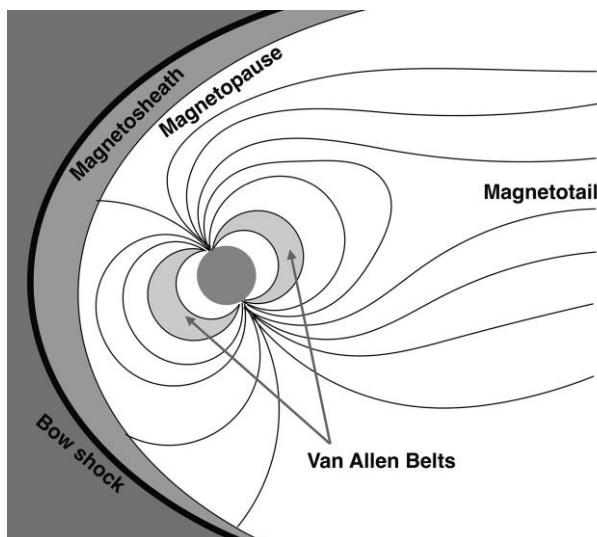
Рисунок 9.1 Магнитное поле Земли. Магнитосфера в значительной степени ограничена солнечным ветром, который создает ударную волну в месте их встречи. Большая часть заряженных частиц не может проникнуть в магнитосферную оболочку непосредственно за ударной волной. Те, которые проникают, обычно находятся в радиационных поясах Ван Аллена и иногда выпадают на магнитные полюса, вызывая полярные сияния.
