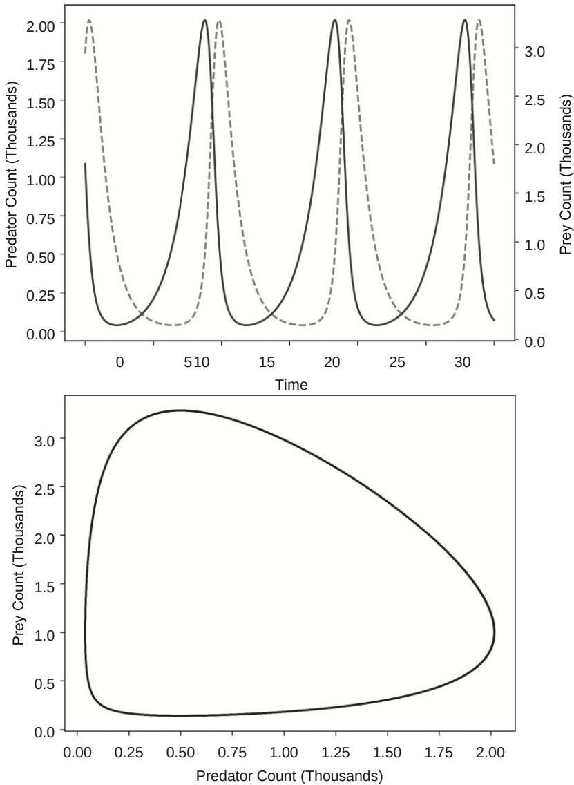
Рисунок 20.1 Динамика взаимодействия хищник-жертва в системе Лотки-Вольтерры. На верхнем графике показана общая численность популяции во времени для системы Лотки-Вольтерры, где \alpha = 1/3 , \beta = 0,666 и \delta = \gamma = 1 . Эволюция обеих популяций носит периодический характер и описывает замкнутую локус в фазовом пространстве R - P (нижний график).
