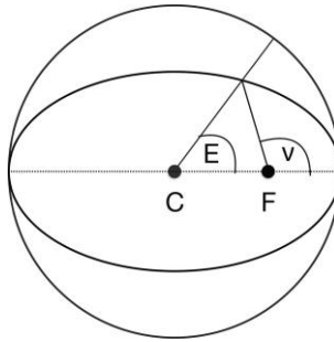
Рисунок 4.2 Эксцентриситет и истинная аномалия кеплеровской орбиты. Тела вращаются по эллипсам вокруг фокуса (F). Эксцентрическая аномалия описывает угол, который вращающееся тело образовывало бы с центром эллипса (C), если бы оно двигалось по круговой орбите. Следовательно, эксцентрическая и истинная аномалия эквивалентны, когда орбита круговая.
