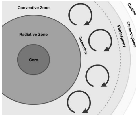
Рисунок 10.1 Внутреннее строение Солнца. Внутри ядра водород превращается в гелий в результате термоядерного синтеза. Две основные зоны звездной атмосферы — радиационная и конвективная — соединены в тахоклине. Фотоны, достигнув фотосферы, свободно вырываются из атмосферы, проходя через горячую хромосферу и за пределы корональной плазмы.
