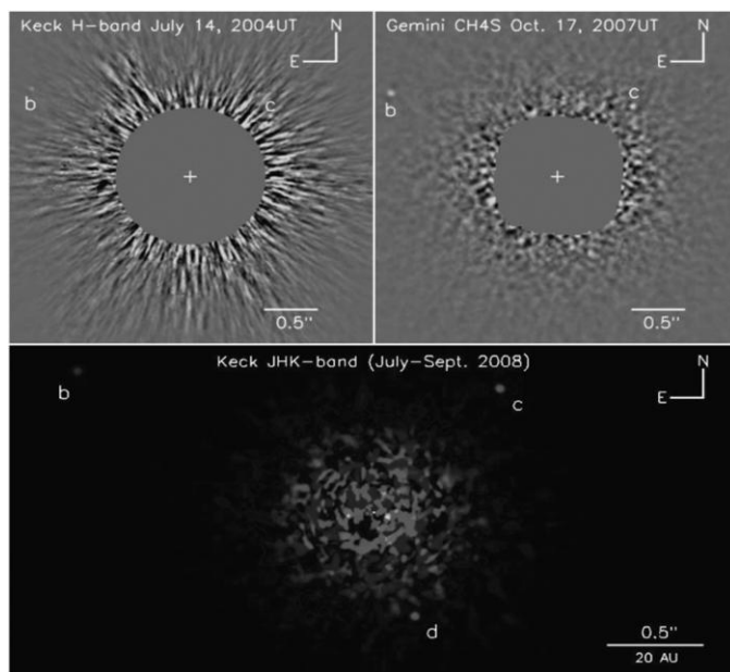
Рисунок 4.7 Обнаружение нескольких экзопланет методом прямой съемки вокруг звезды HR 8799. Артефакты на изображениях вокруг звезды обусловлены методом угловой дифференциации изображения (ADI), используемым для удаления спеклов с изображений. Два верхних изображения представляют собой изображения в одном диапазоне длин волн, а нижнее изображение — трехцветное изображение в трех инфракрасных диапазонах длин волн. Взято из Marois et al. (2008).
