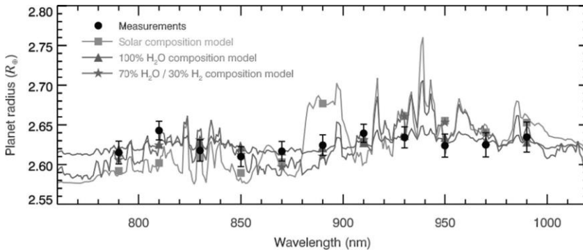
Рисунок 4.4 Спектр суперземли GJ1214b, определенный путем измерения радиуса планеты по данным транзита на нескольких длинах волн. Отсутствие каких-либо особенностей в этом спектре указывает на то, что облачность играет роль заслоняющей силы. Рисунок взят из (Bean et al., 2010).
