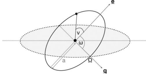
Рисунок 4.1 Кеплеровская орбита. Эллипс орбиты определяется большой полуосью a и эксцентриситетом e . Вектор эксцентриситета e направлен к точке перицентра, а вектор узла \mathbf{q} — к восходящему узлу.
