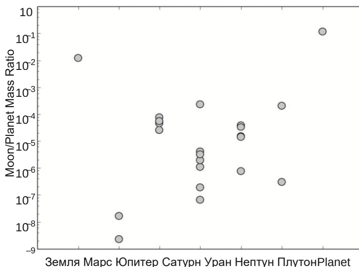
Рисунок 4.13 Соотношение масс лун и планет для основных спутников Солнечной системы. Обратите внимание на различие между Луной Земли и крупнейшим спутником Плутона, Хароном, которые обладают соотношением масс порядка 10^{-2} , и обычными спутниками газовых и ледяных гигантов, у которых соотношение масс порядка 10^{-4} . Данные взяты из базы данных физических параметров планетарных спутников Лаборатории реактивного движения, http://ssd.jpl.nasa.gov
