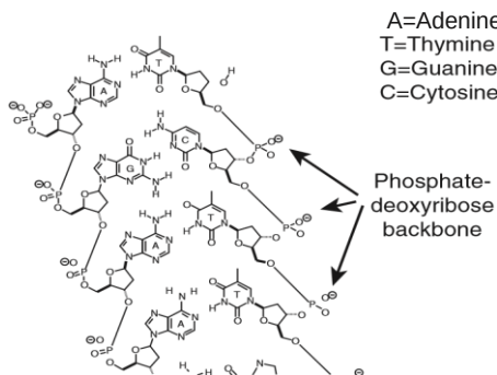
Рисунок 5.4 Химическая структура нити ДНК. Показаны четыре основания ДНК: аденин (А), тимин (Т), гуанин (G) и цитозин (С).
