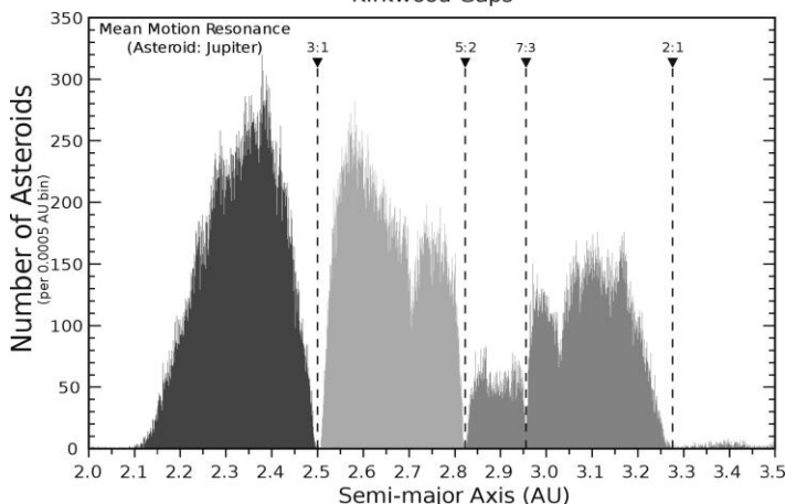
Рисунок 25.1 Пробелы Кирквуда в поясе астероидов. Нестабильные резонансы среднего движения с Юпитером обеспечивают смещение астероидов от определенных больших полуосей орбит. Утверждается, что любой космический аппарат, посещающий пояс астероидов, будет использовать орбиты внутри этих пробелов, чтобы минимизировать риск столкновений. График первоначально предоставлен Аланом Чемберленом, JPL/Caltech. (Gradie et al., 1989)
