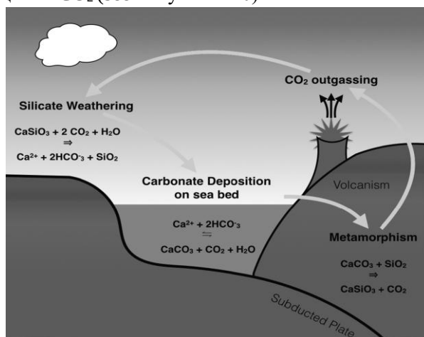
Рисунок 4.10 Карбонатно-силикатный цикл. Парциальное давление атмосферного \text{CO}_2 регулируется образованием угольной кислоты ( \text{H}_2\text{CO}_3 ), которая выветривает силикаты и карбонатные ионы в океан, где они затем включаются в состав морских организмов. После смерти эти организмы возвращаются на морское дно, а карбонаты/силикаты подвергаются субдукции. В результате метаморфизма высвобождается \text{CO}_2 , который возвращается в атмосферу в результате вулканической активности, завершая цикл.
