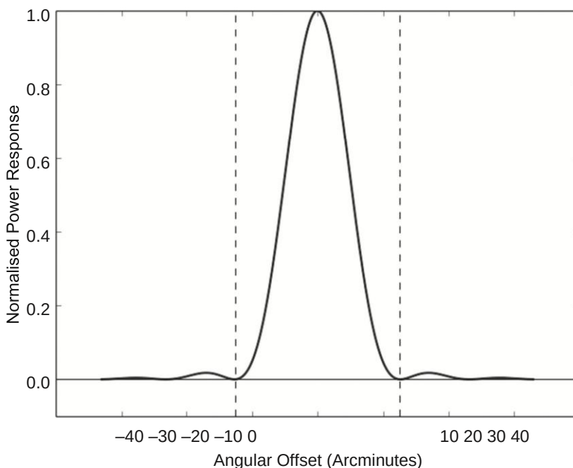
Рисунок 2.7 Зависимость мощности кругового параболического радиотелескопа от смещения относительно центра поля зрения. Первичный луч формируется в пределах 1.22\lambda/D от центра, где мощность равна нулю (обозначено пунктирными линиями). Обратите внимание на боковые лепестки (нормированный пиковый отклик 0.0174) по обе стороны от первичного луча.
