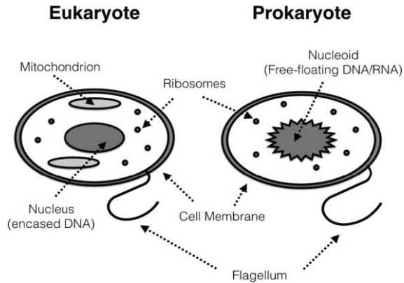
Рисунок 5.5 Упрощенная схема эукариотической и прокариотической клетки. Прокариоты не имеют других органелл, кроме рибосом, мест синтеза белка. Нуклеоид представляет собой совокупность РНК, ДНК и белков, не заключенную в мембрану. В отличие от них, эукариотические клетки имеют ядро, заключенное в мембрану, и множество органелл в зависимости от того, относится ли клетка к растениям или животным. Почти все эукариотические клетки содержат митохондрии, которые производят большую часть запасов аденозинтрифосфата (АТФ) в клетке. Растительные клетки также содержат хлоропласты, которые осуществляют фотосинтез.
