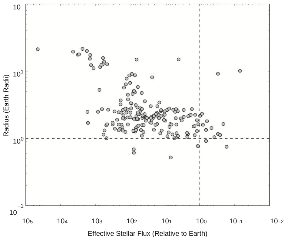
Рисунок 4.9 Радиус экзопланеты (в радиусах Земли) в зависимости от эффективного потока звездного излучения, где 1 = поток звездного излучения, принимаемый Землей. Пунктирные линии показывают значения для Земли. Данные предоставлены Архивом экзопланет НАСА.
