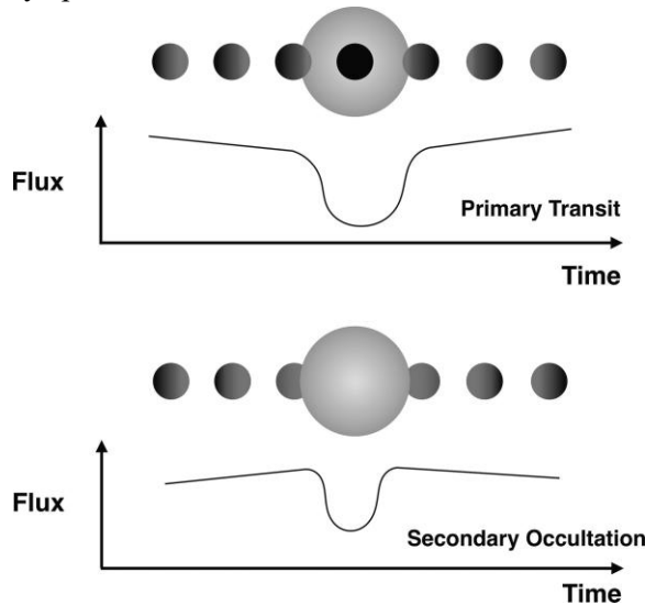
Рисунок 4.3 Транзит планеты по звёздному диску. Первичный транзит (верхний ряд) блокирует небольшую часть света звезды, в то время как затмение или вторичное затмение (нижний ряд) блокирует свет планеты. В промежутках между транзитами и затмениями становятся видимыми небольшие участки поверхности планеты, что приводит к вариациям потока вне транзита (так называемая фазовая кривая).
