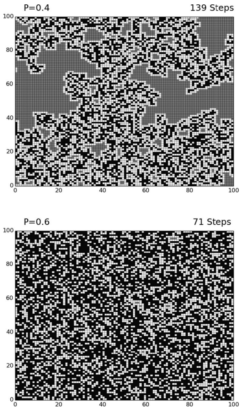
Рисунок 19.1. Примеры перколяционной модели Ландиса (в 2D). Черные квадраты обозначают активные участки колонизации, белые квадраты — участки, колонизация которых прекратилась, а серые квадраты — участки, которые еще не исследованы. Вверху: P = 0,4 , что немного ниже критического значения для 2D квадратных решеток. Видна нитевидная структура участков колонизации, а также большие области неисследованных участков. Внизу: P = 0,6 , что немного выше критического значения, и вся область исследована.
