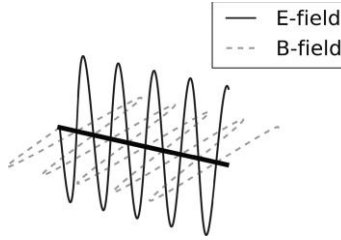
Рисунок 2.2 Электромагнитное поле излучения, состоящее из перпендикулярно колеблющихся электрического и магнитного полей.
