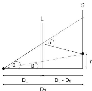
Рисунок 4.5 Геометрия линзирования. Источник (в плоскости источника, обозначенной S) излучает свет, который затем линзируется массой в плоскости линзы L. Затем из этой геометрии выводится уравнение линзирования для определения массы линзы.
