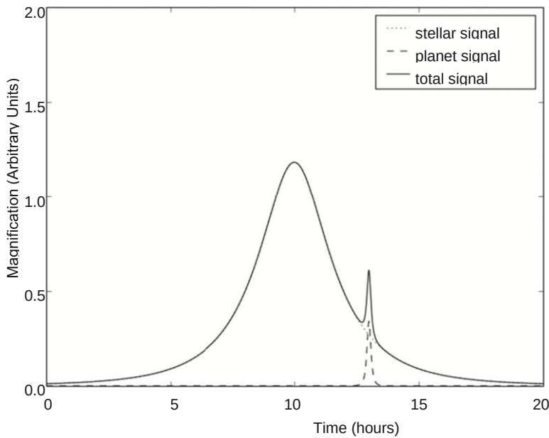
Рисунок 4.6 Характерная кривая блеска, указывающая на событие микролинзирования экзопланеты. Звезда-линза создает главную кривую, причем вклад планеты относительно невелик по амплитуде и исключительно кратковременный.
