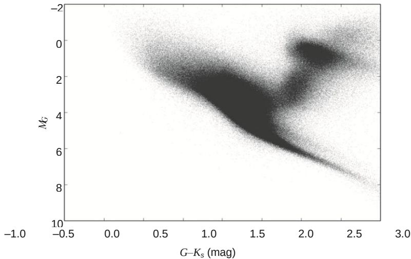
Рисунок 10.2 Диаграмма Герцшпрунга-Рассела, построенная на основе данных Gaia Data Release 1. Обратите внимание, что эффективная температура (ось x, где в качестве показателя используется спектральный цвет) увеличивается справа налево. Большинство звезд расположены вдоль главной последовательности (центральная полоса), а более развитые звезды перемещаются в верхнюю правую часть диаграммы. Источник: ESO
