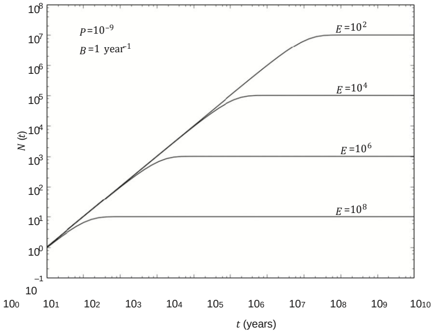
Рисунок 14.1 Число цивилизаций, способных к взаимодействию, как функция времени, при условии, что E индивидов вызывают самоуничтожение с вероятностью P на одного индивида в год. Скорость рождаемости цивилизаций B фиксирована на уровне одного индивида в год.
