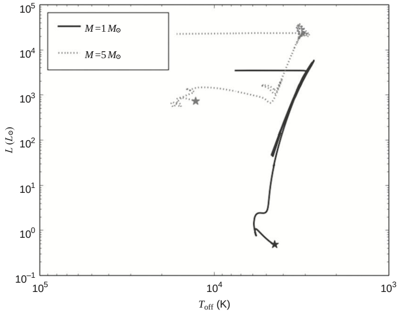
Рисунок 10.3 Эволюция звезды массой 1M (сплошная линия) и звезды массой 5M (пунктирная линия) на диаграмме Герцшпрунга. Мы начинаем движение с обеих звезд на главной последовательности (через ветвь субгигантов к ветви красных гигантов (RGB)). Звезда массой 1M эволюционирует вдоль главной последовательности и, начиная с главной последовательности, начинает термоядерный синтез гелия в своем ядре, затем опускается вниз и присоединяется к асимптотической ветви гигантов (AGB), которая точно следует за RGB. Достигнув вершины AGB (когда горение гелия в ядре прекращается), звезда эволюционирует в сторону фазы планетарной туманности/белого карлика (не показано на графике). Звезда массой 5M быстро перескакивает через «синюю петлю», прежде чем присоединиться к AGB, поскольку она способна начать термоядерный синтез гелия в углерод еще до того, как покинет RGB. Данные получены в рамках проекта MESA Isochrones and Stellar Tracks с использованием кода MESA для моделирования эволюции звезд.
