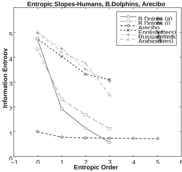
Рисунок 21.5 Информационная энтропия как функция энтропийного порядка (Рисунок 4а из работы Doyle et al., 2011). Обратите внимание, что английский, русский и арабский языки, как правило, следуют закону Ципфа с показателем степенного закона -1 . Сообщение из Аресибо не демонстрирует сильных условных связей между битами, поэтому энтропия относительно постоянна на всех порядках. Дельфины-афалины также демонстрируют синтаксическую структуру в своей коммуникации благодаря убывающей энтропии с порядком.
