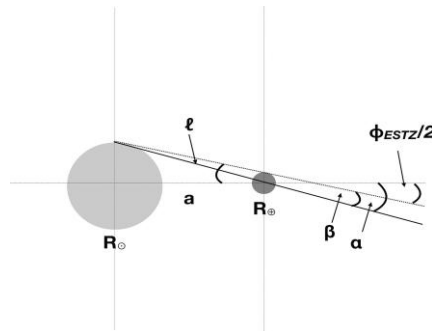
Рисунок 27.1 Транзитная зона Земли, определяемая как угловая область \phi_{ESTZ} = 2(\alpha - \beta) \sim R/a в пределах R \gg R_{\oplus} .
