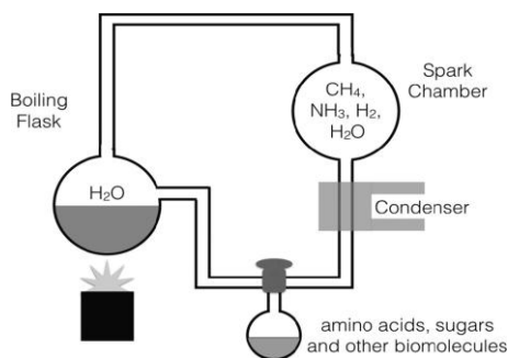
Рисунок 5.2 Схема эксперимента Миллера-Урея. Вода испарялась и добавлялась в искровую камеру, содержащую вещества, которые, как предполагалось, присутствовали в атмосфере ранней Земли. Через эту камеру пропусклся электрический разряд, а продукты конденсировались и собирались для изучения. В результате этого эксперимента были получены как аминокислоты, так и предшественники нуклеотидов RNA и DNA.
