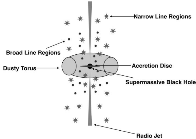
Рисунок 11.1 Стандартная унифицированная модель активных галактических ядер (AGN). Центральная черная дыра окружена аккреционным диском размером в несколько сотен астрономических единиц, который заключен в пылевой тор. Этот тор пронизан мощными радиоджетами и ветрами, исходящими от черной дыры, которые освещают широкие и узкие области эмиссионных линий, причем ширина эмиссионных линий, исходящих из этих областей, сильно зависит от их расстояния от черной дыры (и, как следствие, от их орбитальной скорости вокруг нее).
