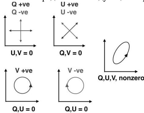
Рисунок 2.3 Схема различных форм поляризации с соответствующими значениями параметров Стокса ( I, Q, U, V ).
