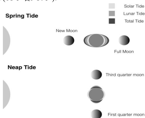
Рисунок 4.14 Весенние и отливные приливы. В зависимости от относительной ориентации Солнца и Луны, лунные и солнечные приливы могут суммироваться, образуя весенний прилив, или суммироваться перпендикулярно, образуя отливной прилив.
