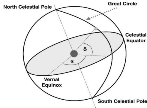
Рисунок 2.1 Экваториальная система координат. Небесная сфера определяется небесным экватором (плоскостью, содержащей экватор Земли), небесными северным и южным полюсами, перпендикулярными этой плоскости, и контрольным местоположением на экваторе (точка весеннего равноденствия). Затем с помощью этой системы можно рассчитать прямое восхождение \alpha и склонение \delta с соответствующим расчетом часового угла, который учитывает вращение Земли.
