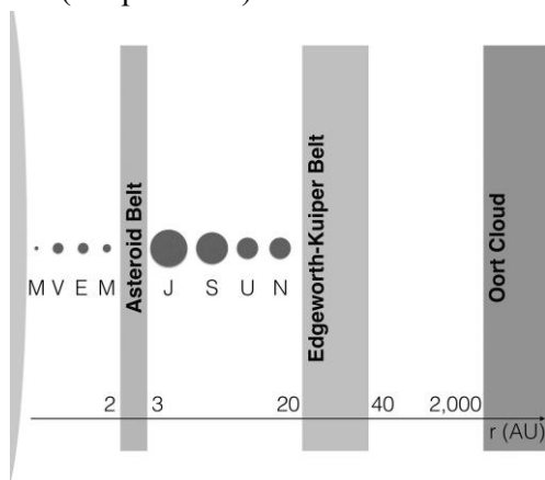
Рисунок 4.12 Положения основных семейств астероидов и комет в Солнечной системе относительно восьми известных планет..
