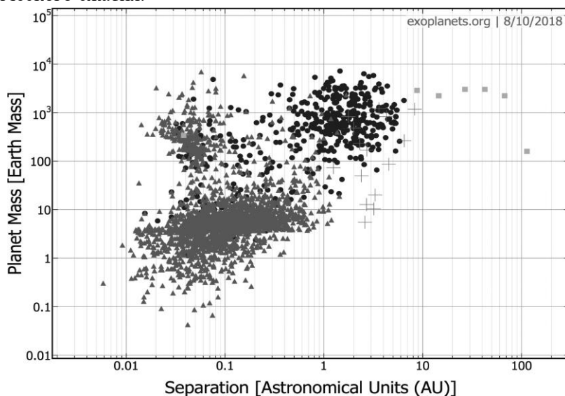
Рисунок 4.8 Зависимость количества экзопланет от массы планеты и большой полуоси орбиты, полученная с помощью Exoplanet Data Explorer (exoplanets.org, доступ от 10 августа 2018 г.). Треугольники обозначают экзопланеты, обнаруженные транзитом, круги — обнаруженные методом радиальной скорости, кресты — методом микролинзирования, а квадраты — методом прямого изображения.
