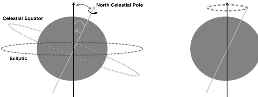
Рисунок 4.11 Наклон оси Земли \delta_0 . С наклоном оси связаны два цикла Миланковича. В первом цикле величина наклона оси может изменяться (слева). Во втором цикле наклон оси прецессирует (справа)
