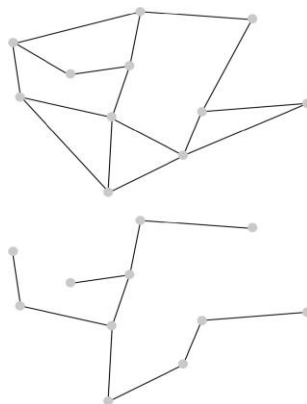
Рисунок 22.1 Вверху: Пример полностью связного графа, состоящего из вершин (круги) и ребер (линии). Внизу: Минимальное остовное дерево того же графа.
