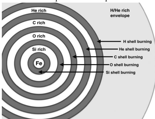
Рисунок 10.4 «Лукообразная» структура звезды с массой более 800 мкг/м³ состоит из различных элементов, подвергающихся «сжиганию оболочек», которые затем сливаются, образуя следующий слой. Элементы располагаются в последовательности H, He, C, O, Si, Fe (другие элементы встречаются в относительно небольших количествах). Железо не может быть успешно синтезировано, поскольку реакция синтеза становится эндотермической.
