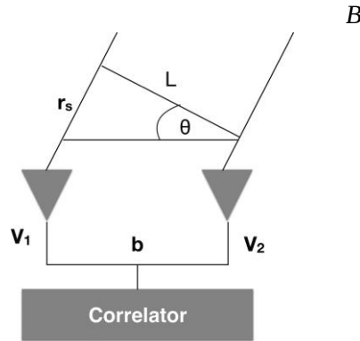
Рисунок 2.8 Схема двухэлементного интерферометра. Сигналы попадают на оба детектора с временной задержкой, определяемой разностью хода L . Затем напряжения, индуцированные в обоих детекторах, коррелируются, образуя единственную фурье-компоненту распределения яркости неба.
