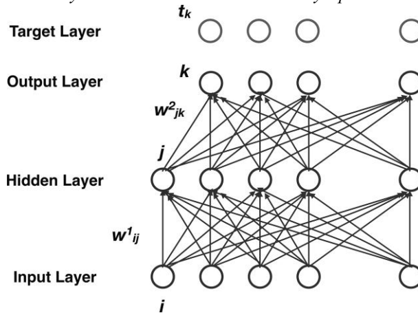
Рисунок 15.2 Трехслойная нейронная сеть обратного распространения ошибки. Каждый нейрон i во входном слое соединен со скрытым слоем с помощью веса соединения w_{ij}^1 . Затем каждый нейрон в скрытом слое соединен с нейроном в выходном слое k с помощью веса w_{jk}^2 . Выходы x_k сравниваются с целевыми выходами t_k .
