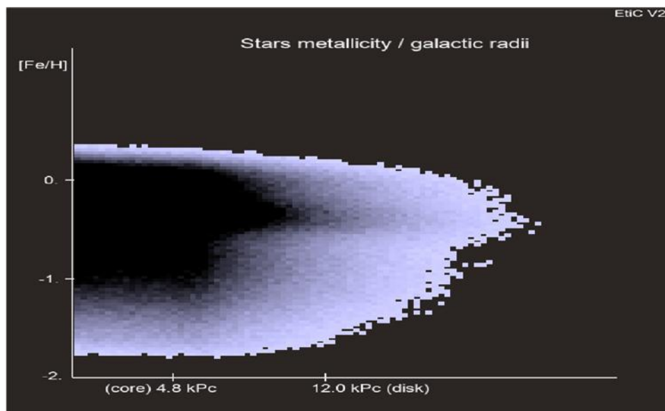
Рис. 13 – Металличность звёзд как функция галактического радиуса
