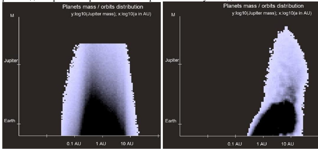
Рисунок 18. Распределение планет по большим полуосям справа: вариант "Акрет", ниже: "масштабированная модель Титуса-Боде"
