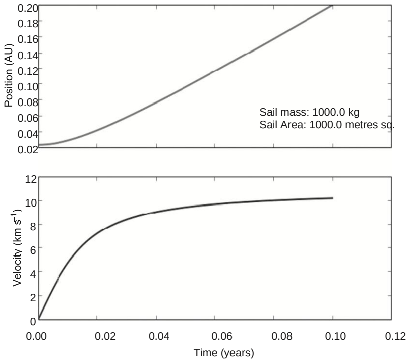
Рисунок 19.4 Изменение положения и скорости солнечного паруса массой 1 тонна (площадь 1000 \text{ м}^2 ) по мере его ускорения при удалении от Солнца, начиная с расстояния в 5 солнечных радиусов.
