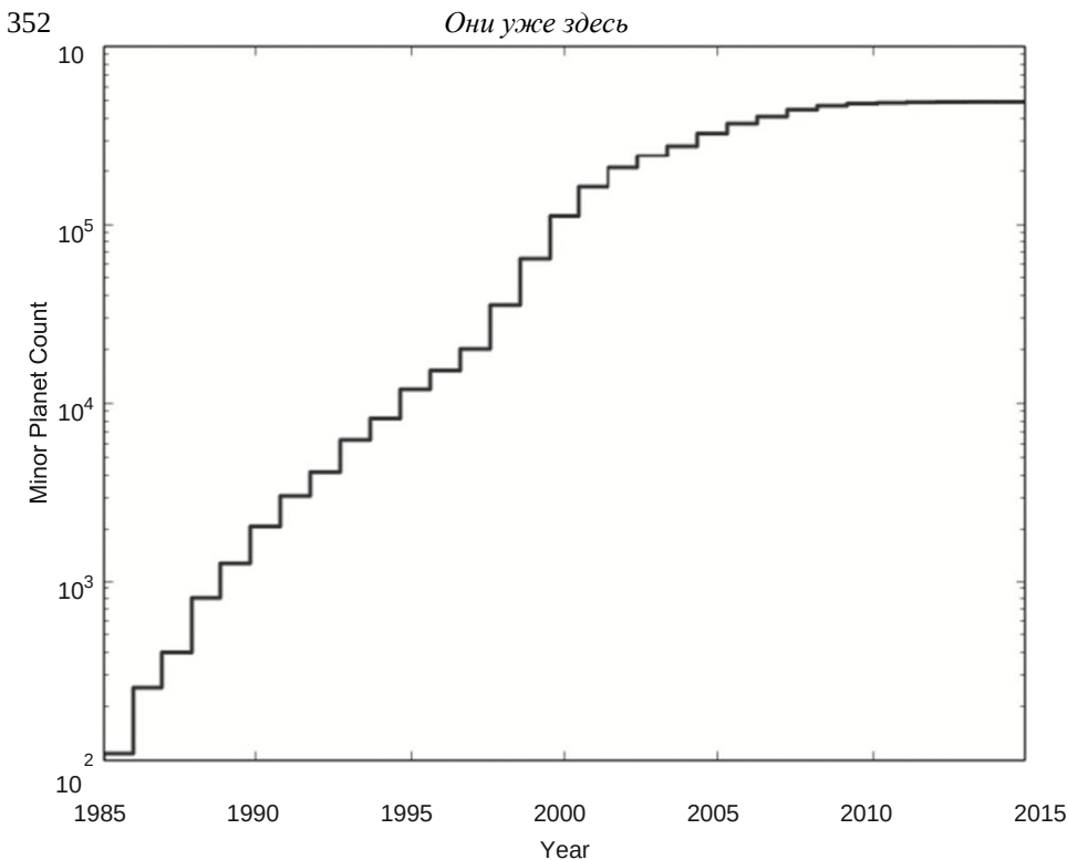
Рисунок 25.2 Общее количество зарегистрированных малых планет (астероидов, комет и карликовых планет) в зависимости от времени. За последние несколько десятилетий было обнаружено чрезвычайно большое количество таких объектов. Данные предоставлены Центром малых планет Международного астрономического союза.
