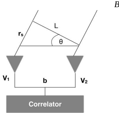
Рисунок 2.8 Схема двухэлементного интерферометра. Сигналы попадают на оба детектора с временной задержкой, определяемой разностью хода $L$. Затем напряжения, индуцированные в обоих детекторах, коррелируются, образуя единственную фурье-компоненту распределения яркости неба.
