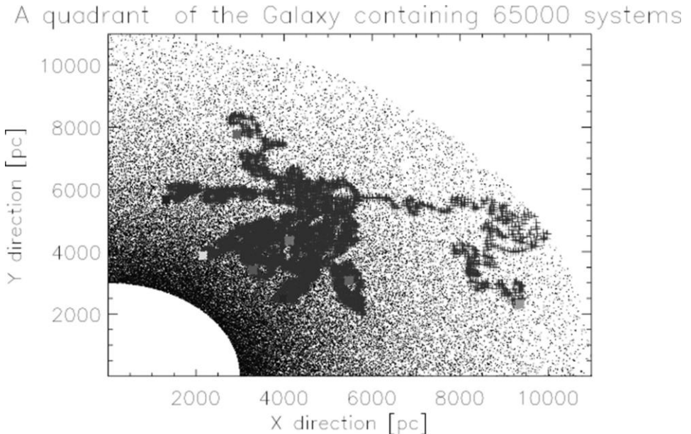
Рисунок 19.2 Пример исследования зонда в симуляциях Бьорка (Björk, 2007).
