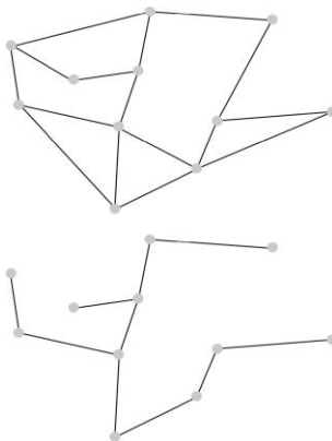
Рисунок 22.1 Вверху: Пример полностью связного графа, состоящего из вершин (круги) и ребер (линии). Внизу: Минимальное остоное дерево того же графа.
