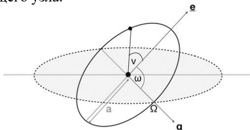
Рисунок 4.1 Кеплеровская орбита. Эллипс орбиты определяется большой полуосью a и эксцентриситетом e . Вектор эксцентриситета \mathbf{e} направлен к точке перицентра, \mathbf{a} — к восходящему узлу.
