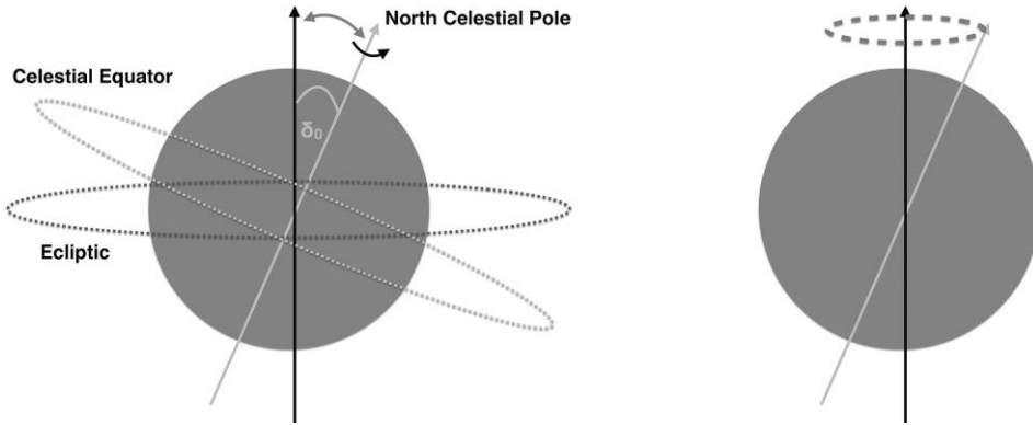
Рисунок 4.11 Наклон оси Земли \delta_0 . С наклоном оси связаны два цикла Миланковича. В первом цикле величина наклона оси может изменяться (слева). Во втором цикле наклон оси прецессирует (справа)
