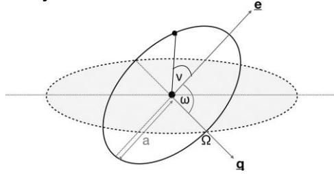
Рисунок 4.1 Кеплеровская орбита. Эллипс орбиты определяется большой полуосью a и эксцентриситетом e . Вектор эксцентриситета e направлен к точке перицентра, а вектор узла q — к восходящему узлу.
