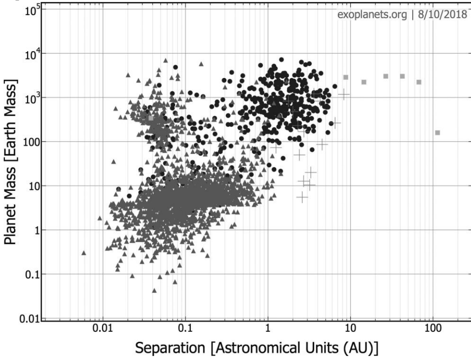
Рисунок 4.8 Зависимость количества экзопланет от массы планеты и большой полуоси орбиты, полученная с помощью Exoplanet Data Explorer (exoplanets.org, доступ от 10 августа 2018 г.). Треугольники обозначают экзопланеты, обнаруженные транзитом, круги — обнаруженные методом радиальной скорости, кресты — методом микролинзирования, а квадраты — методом прямого изображения.
