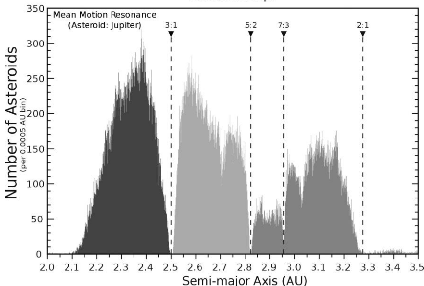
Рисунок 25.1 Пробелы Кирквуда в поясе астероидов. Нестабильные резонансы среднего движения с Юпитером обеспечивают смещение астероидов от определенных больших полуосей орбит. Утверждается, что любой космический аппарат, посещающий пояс астероидов, будет использовать орбиты внутри этих пробелов, чтобы минимизировать риск столкновений. График первоначально предоставлен Аланом Чемберленом, JPL/Caltech. (Gradie et al., 1989)
