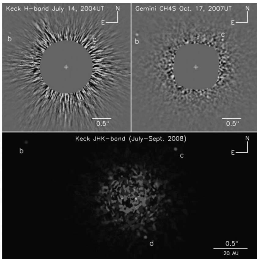
Рисунок 4.7 Обнаружение нескольких экзопланет методом прямой съемки вокруг звезды HR 8799. Артефакты на изображении вокруг звезды обусловлены методом угловой дифференциации изображения (ADI), используемым для удаления спеклов с изображений. Два верхних изображения представляют собой изображения в одном диапазоне длин волн, а нижнее изображение — трехцветное изображение в трех инфракрасных диапазонах длин волн. Взято из Marois et al. (2008).
