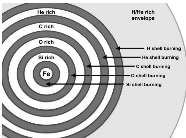
Рисунок 10.4 «Лукообразная» структура звезды с массой более 800 \text{ мкг/м}^3 состоит из различных элементов, подвергающихся «сжиганию оболочек», которые затем сливаются, образуя следующий слой М. Элементы располагаются в последовательности H, He, C, O, Si, Fe (другие элементы встречаются в относительно небольших количествах). Железо не может быть успешно синтезировано, поскольку реакция синтеза становится эндотермической.
