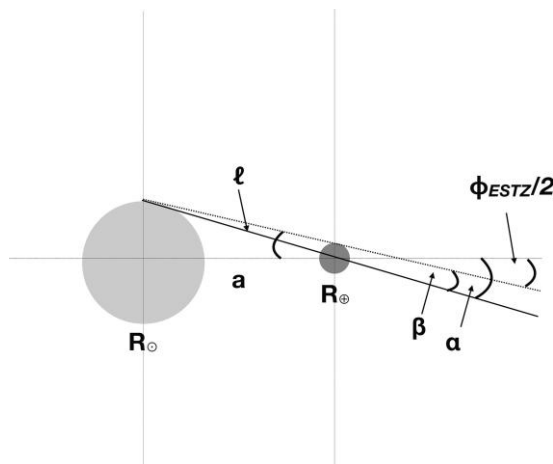
Рисунок 27.1 Транзитная зона Земли, определяемая как угловая область \phi_{ESTZ} = 2(\alpha - \beta) \sim R_{\odot}/a в пределах R \gg R_{\oplus} .
