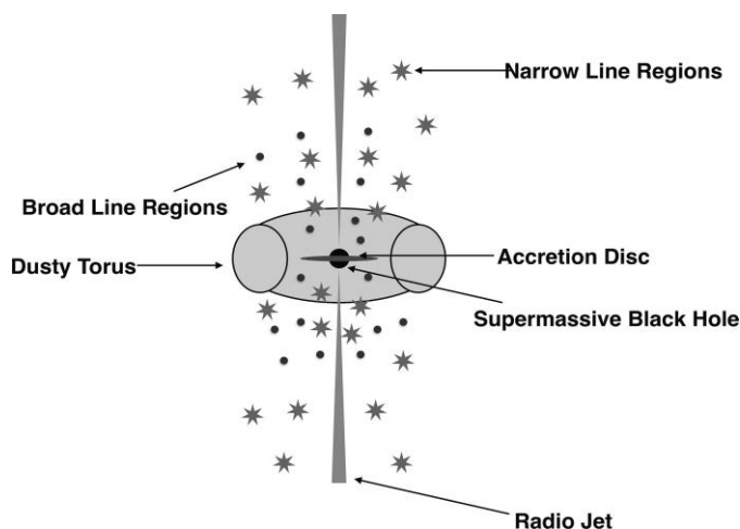
Рисунок 11.1 Стандартная унифицированная модель активных галактических ядер (АГЯ). Центральная черная дыра окружена аккреционным диском размером в несколько сотен астрономических единиц, который заключен в пылевой тор. Этот тор пронизан мощными радиоджетами и ветрами, исходящими от черной дыры, которые освещают широкие и узкие области эмиссионных линий, причем ширина эмиссионных линий, исходящих из этих областей, сильно зависит от их расстояния от черной дыры (и, как следствие, от их орбитальной скорости вокруг нее)..
