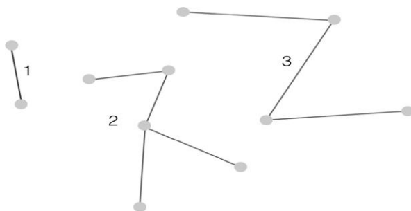
Рисунок 22.2 Пример графа с тремя связными компонентами.
