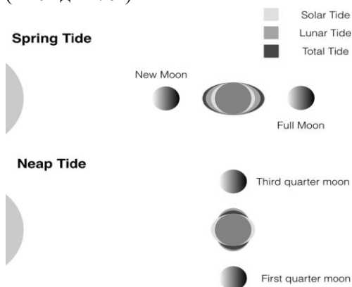
Рисунок 4.14 Весенние и отливные приливы. В зависимости от относительной ориентации Солнца и Луны, лунные и солнечные приливы
