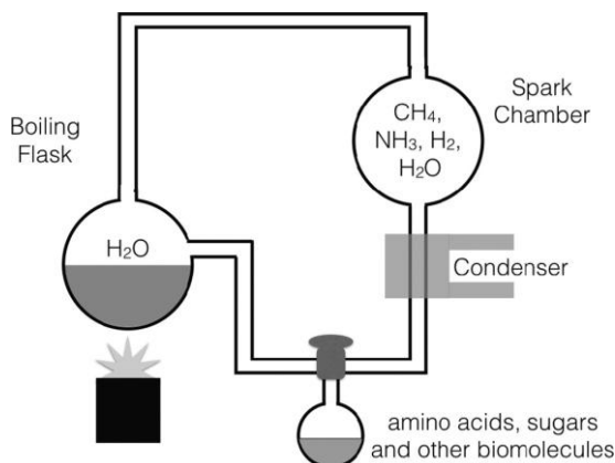
Рисунок 5.2 Схема эксперимента Миллера-Урея. Вода испарялась и добавлялась в искровую камеру, содержащую вещества, которые, как предполагалось, присутствовали в атмосфере ранней Земли. Через эту камеру пропускался электрический разряд, а продукты конденсировались и собирались для изучения. В результате этого эксперимента были получены как аминокислоты, так и предшественники нуклеотидов RNA и DNA.
