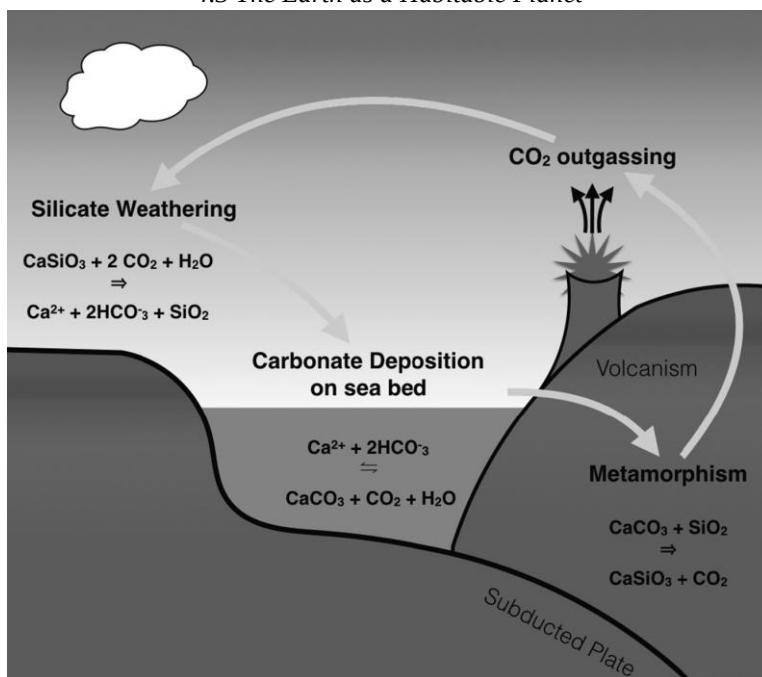
Рисунок 4.10 Карбонатно-силикатный цикл. Парциальное давление атмосферного \text{CO}_2 регулируется образованием угольной кислоты ( \text{H}_2\text{CO}_3 ), которая выветривает силикаты и карбонатные ионы в океан, где они затем включаются в состав морских организмов. После смерти эти организмы возвращаются на морское дно, а карбонаты/силикаты подвергаются субдукции. В результате метаморфизма высвобождается \text{CO}_2 , который возвращается в атмосферу в результате вулканической активности, завершая цикл.
