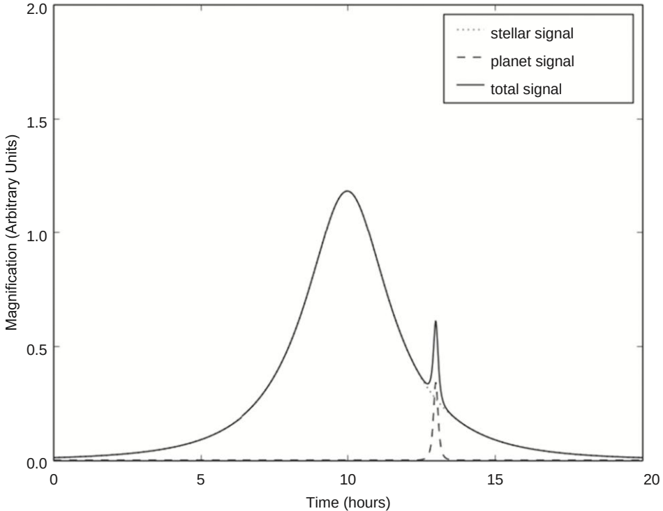
Рисунок 4.6 Характерная кривая блеска, указывающая на событие микролинзирования экзопланеты. Звезда-линза создает главную кривую,
