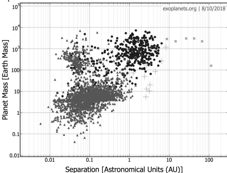
Рисунок 4.8 Зависимость количества экзопланет от массы планеты и большой полуоси орбиты, полученная с помощью Exoplanet Data Explorer (exoplanets.org, доступ от 10 августа 2018 г.). Треугольники обозначают экзопланеты, обнаруженные транзитом, круги — обнаруженные методом радиальной скорости, кресты — методом микролинзирования, а квадраты — методом прямого изображения.
