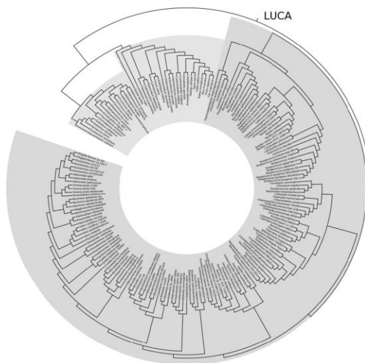
Рисунок 5.1 Филогенетическое Дерево жизни с общими доменами жизни, начиная с верхнего левого угла и по часовой стрелке: археи, эукариоты и бактерии. Последний общий универсальный предок (LUCA) представлен выемкой в правом верхнем углу самой внешней границы. Это дерево было сгенерировано с помощью инструмента iTOL (Letunic and Bork, 2016).
