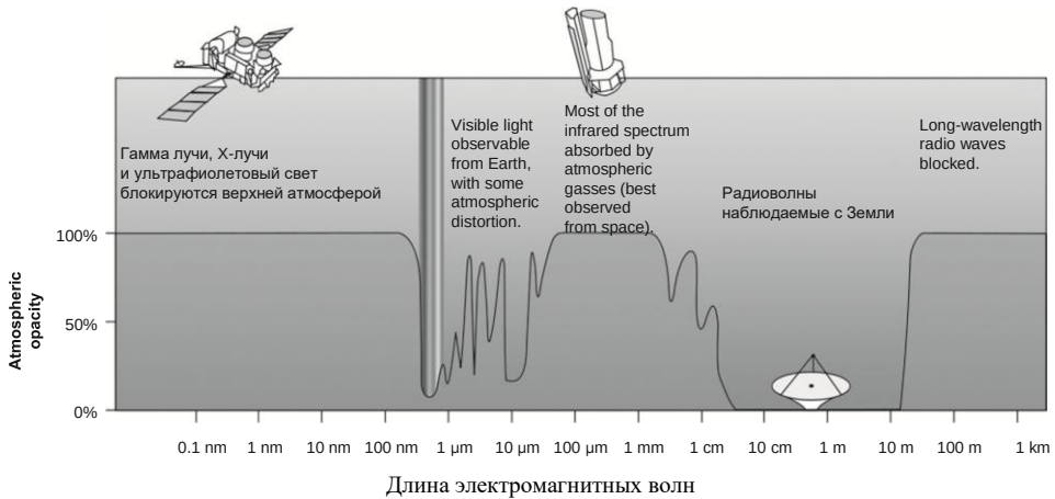
Рисунок 2.4 Атмосферная непрозрачность как функция длины волн. Области с низкой непрозрачностью подходят для наземной астрономии. Радиоизлучение в диапазоне от 1 см до 10 м хорошо наблюдается с поверхности Земли. (Источник оригинального изображения: NASA)
