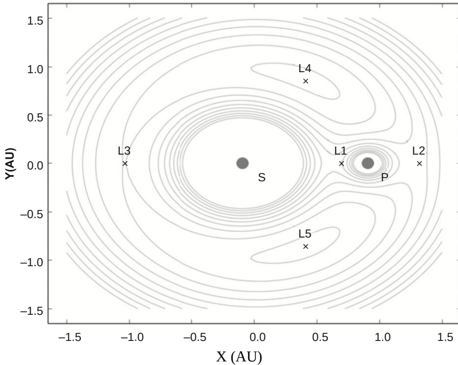
Рисунок 4.15 Точки Лагранжа системы звезда-планета (в системе отсчета, вращающейся вместе с планетой). Для иллюстрации масса планеты (P) составляет одну десятую массы звезды (S). Контурные обозначают эквипотенциальные поверхности, вычисленные на основе эффективного потенциала гравитации звезды и планеты, а также центробежной силы. L1, L2 и L3 являются номинально неустойчивыми точками (максимумами потенциала), хотя вокруг них можно успешно вращаться с минимальным поддержанием положения. L4 и L5 являются устойчивыми (минимумами потенциала). Предполагается, что Луна могла образоваться в одной из точек L4 или L5 Земли.
