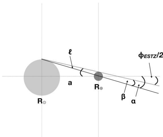
Рисунок 27.1 Транзитная зона Земли, определяемая как угловая область \phi_{ESTZ} = 2(\alpha - \beta) \sim R_{\odot}/a в пределах R \gg R_{\oplus} .
