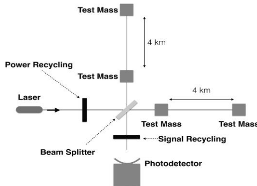
Рисунок 21.3 Упрощенная схема установки LIGO, которая в 2015 году успешно зарегистрировала гравитационные волны от слияния черных дыр звездной массы.
