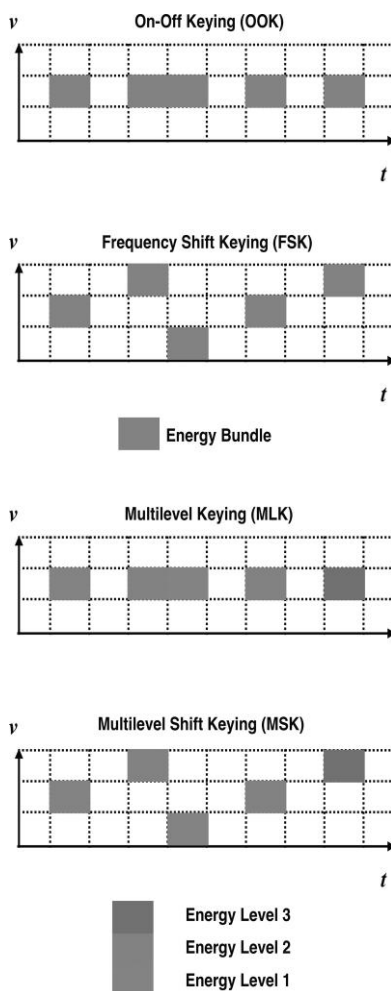
Рисунок 21.1 Спектрально и энергоэффективные схемы кодирования. На каждом графике представлены энергетические пакеты (блоки), передаваемые на определенной частоте \nu в момент времени t . В первом случае — манипуляция «вкл.-выкл.» (OOK), а во втором — частотная манипуляция (FSK), использующие одну фиксированную энергию пакета. Внизу: многоуровневая манипуляция (MLK), поддерживающая спектральную эффективность за счет передачи диапазона M энергий пакетов. В данном случае M = 3 , что дает \log 23 = 1.58 бит информации на пакет; и многоуровневая манипуляция (MSK), сочетающая в себе преимущества (и недостатки) как MLK, так и FSK.
