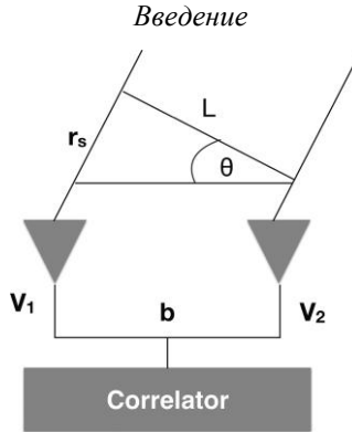
Рисунок 2.8 Схема двухэлементного интерферометра. Сигналы попадают на оба детектора с временной задержкой, определяемой разностью хода L . Затем напряжения, индуцированные в обоих детекторах, коррелируются, образуя единственную фурье-компоненту распределения яркости неба.
