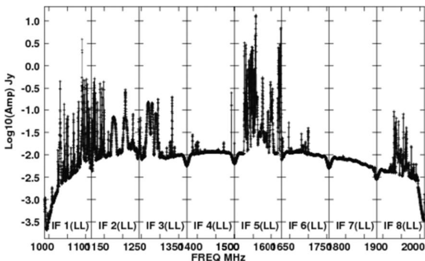
Рисунок 2.6 Радиочастотные помехи (РЧП), измеренные на радиотелескопе Very Large Array в Нью-Мексико в L-диапазоне (1–2 ГГц). Пики в приведенном выше спектре указывают на сигналы от таких источников, как спутники GPS и метеорологические спутники, радиолокационные импульсы от близлежащих установок и передачи модемов на площадке VLA. Данные предоставлены NRAO.
