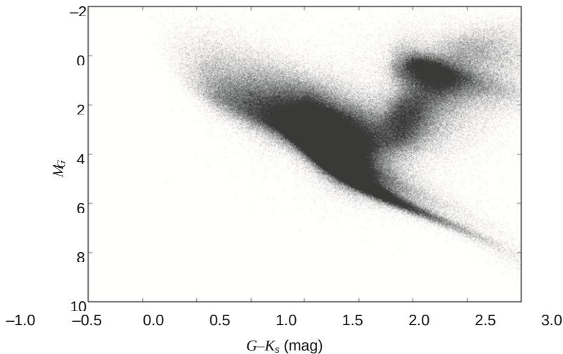
Рисунок 10.2 Диаграмма Герцшпрунга-Рассела, построенная на основе данных Gaia Data Release 1. Обратите внимание, что эффективная температура (ось x , где в качестве показателя используется спектральный цвет) увеличивается справа налево. Большинство звезд расположены вдоль главной последовательности (центральная полоса), а более развитые звезды перемещаются в верхнюю правую часть диаграммы. Источник: ESO
