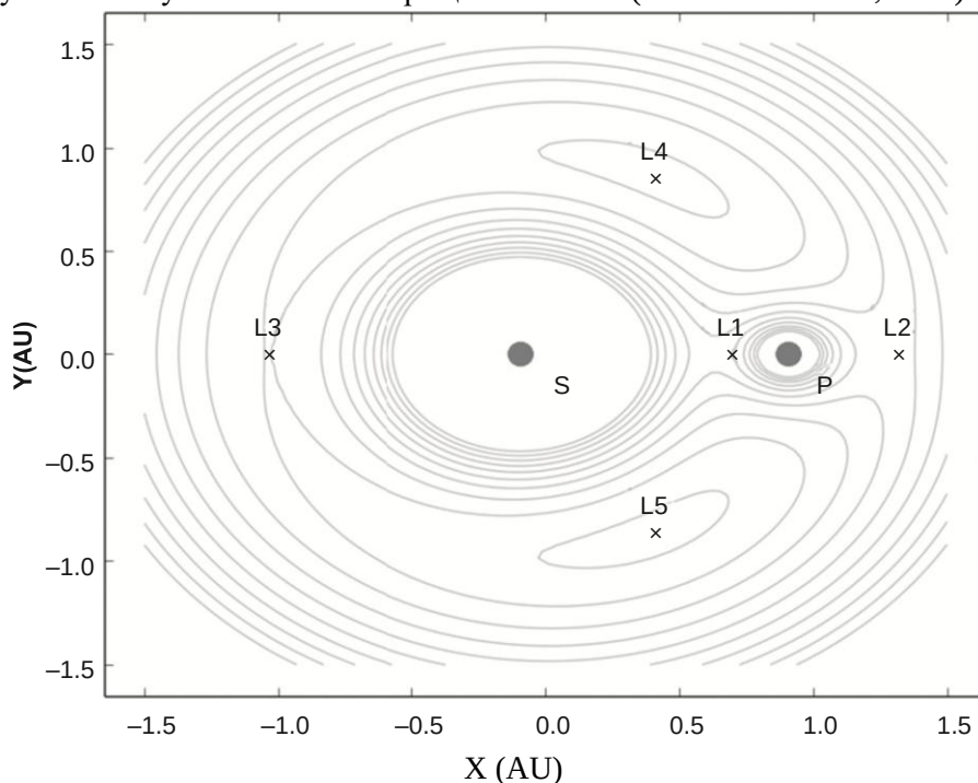
Рисунок 4.15 Точки Лагранжа системы звезда-планета (в системе отсчета, вращающейся вместе с планетой). Для иллюстрации масса планеты (P) составляет одну десятую массы звезды (S). Контуры обозначают эквипотенциальные поверхности, вычисленные на основе эффективного потенциала гравитации звезды и планеты, а также центробежной силы. L1, L2 и L3 являются номинально неустойчивыми точками (максимумами потенциала), хотя вокруг них можно успешно вращаться с минимальным поддержанием положения. L4 и L5 являются устойчивыми (минимумами потенциала). Предполагается, что Луна могла образоваться в одной из точек L4 или L5 Земли.
