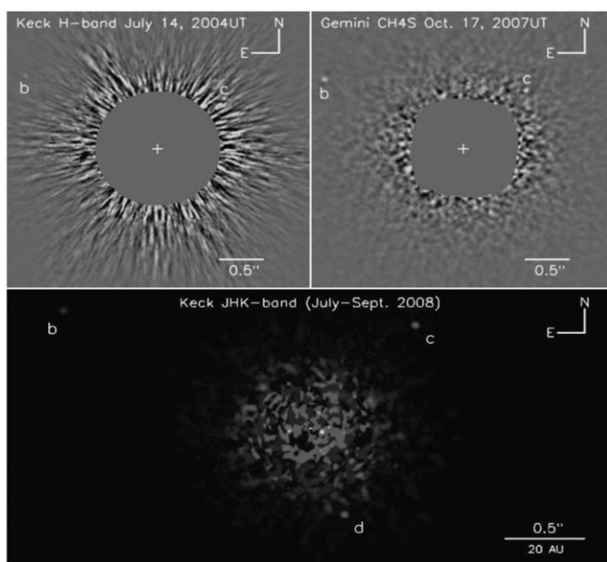
Рисунок 4.7 Обнаружение нескольких экзопланет методом прямой съемки вокруг звезды HR 8799. Артефакты на изображении вокруг звезды обусловлены методом угловой дифференциации изображения (ADI), используемым для удаления спеклов с изображений. Два верхних изображения представляют собой изображения в одном диапазоне длин волн, а нижнее изображение — трехцветное изображение в трех инфракрасных диапазонах длин волн. Взято из Marois et al. (2008).
