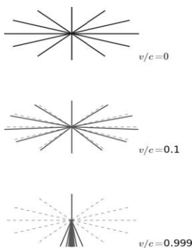
Рисунок 19.7 Иллюстрация релятивистской абберации. Свет излучается источниками, находящимися в состоянии покоя, вдоль радиальных линий зрения в направлении нашего космического аппарата, также находящегося в состоянии покоя (верхний рисунок). Источники, расположенные немного позади этих точек, будут по-прежнему видны наблюдателю, движущемуся на космическом аппарате со скоростью 0,1c (средний рисунок). При высоких релятивистских скоростях поле зрения наблюдателя приближается к 360^\circ (нижний рисунок).
