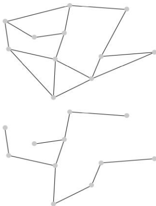
Рисунок 22.1 Вверху: Пример полностью связного графа, состоящего из вершин (круги) и ребер (линии). Внизу: Минимальное остоное дерево того же графа.
