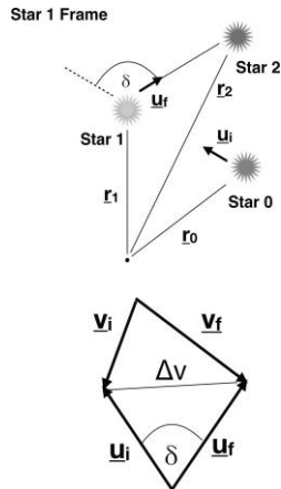
Рисунок 19.6 Гравитационный маневр, или гравитационный маневр. Вверху: Гравитационный маневр в системе отсчета звезды 1. Начиная от звезды 0, зонд достигает скорости u_i в системе отсчета звезды 1 и покидает звезду 1, двигаясь к звезде 2 со скоростью u_f , имеющей ту же величину. Внизу: Сравнение скоростей в лабораторной системе отсчета ( v_i, v_f ) к скорости в системе отсчета звезды 1.
