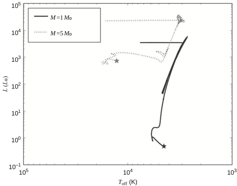
Рисунок 10.3 Эволюция звезды массой 1М (сплошная линия) и звезды массой 5М (пунктирная линия) на диаграмме Герцшпрунга. Мы начинаем движение с обеих звезд на главной последовательности (через ветвь субгигантов к ветви красных гигантов (RGB)). Звезда массой 1М эволюционирует вдоль главной последовательности и, начиная с главной последовательности, начинает термоядерный синтез гелия в своем ядре, затем опускается вниз и присоединяется к асимптотической ветви гигантов (AGB), которая точно следует за RGB. Достигнув вершины AGB (когда горение гелия в ядре прекращается), звезда эволюционирует в сторону фазы планетарной туманности/белого карлика (не показано на графике). Звезда массой 5М быстро перескакивает через «синюю петлю», прежде чем присоединиться к AGB, поскольку она способна начать термоядерный синтез гелия в углерод еще до того, как покинет RGB. Данные получены в рамках проекта MESA Isochrones and Stellar Tracks с использованием кода MESA для моделирования эволюции звезд.
