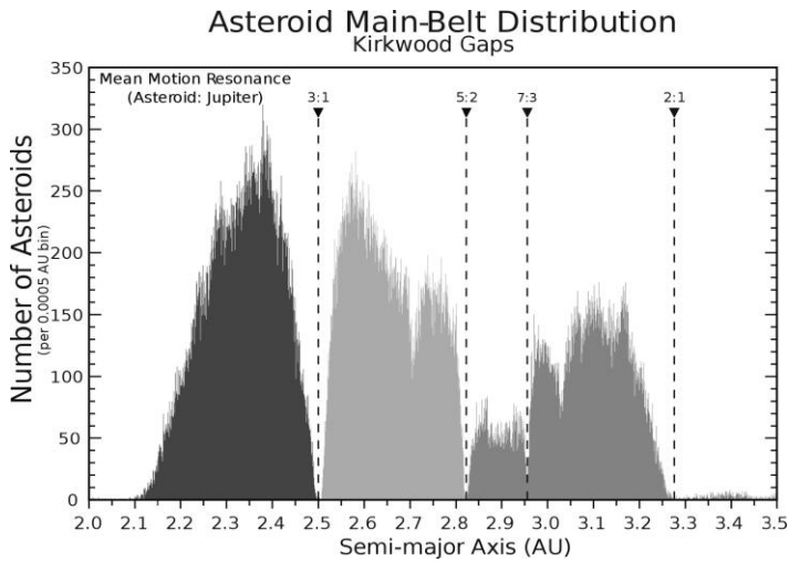
Рисунок 25.1 Пробелы Кирквуда в поясе астероидов. Нестабильные резонансы среднего движения с Юпитером обеспечивают смещение астероидов от определенных больших полуосей орбит. Утверждается, что любой космический аппарат, посещающий пояс астероидов, будет использовать орбиты внутри этих пробелов, чтобы минимизировать риск столкновений. График первоначально предоставлен Аланом Чемберленом, JPL/Caltech. (Gradie et al., 1989)
