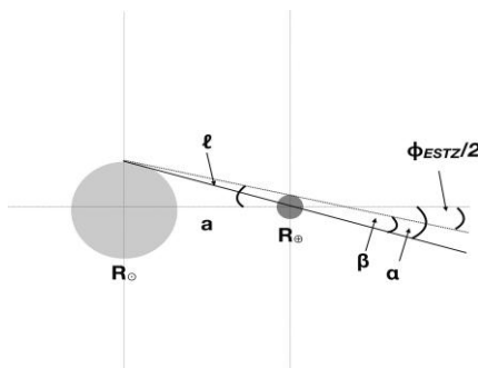
Рисунок 27.1 Транзитная зона Земли, определяемая как угловая область \phi_{ESTZ} = 2(\alpha - \beta) \sim R_{\oplus}/a в пределах R \gg R_{\oplus} .
