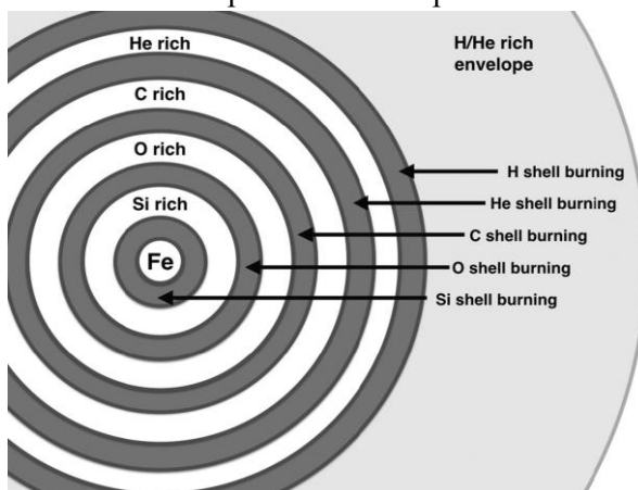
Рисунок 10.4 «Лукообразная» структура звезды с массой более 800 \text{ мкг/м}^3 состоит из различных элементов, подвергающихся «сжиганию оболочек», которые затем сливаются, образуя следующий слой. Элементы располагаются в последовательности H, He, C, O, Si, Fe (другие элементы встречаются в относительно небольших количествах). Железо не может быть успешно синтезировано, поскольку реакция синтеза становится эндотермической.
