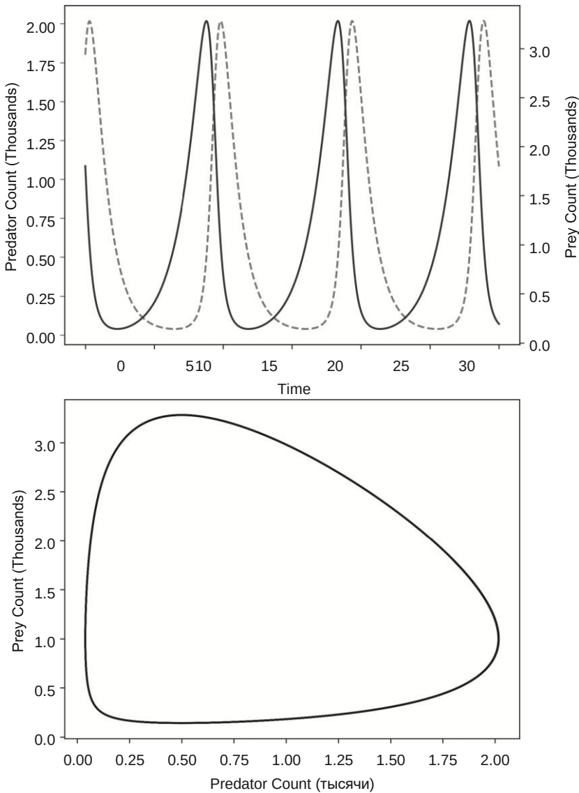
Рисунок 20.1 Динамика взаимодействия хищник-жества в системе Лотки-Вольтерры. На верхнем графике показана общая численность популяции во времени для системы Лотки-Вольтерры, где \alpha = 1/3 , \beta = 0,666 и \delta = \gamma = 1 . Эволюция обеих популяций носит периодический характер и описывает замкнутую локус в фазовом пространстве R – P (нижний график).
