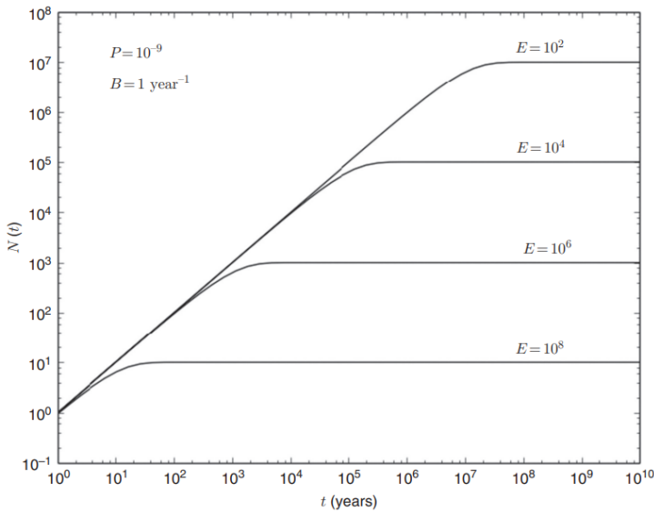
Рисунок 14.1 Число коммуникативных цивилизаций как функция времени, при условии, что E индивидов вызывают самоуничтожение с вероятностью P на одного индивида в год. Скорость возникновения цивилизаций B фиксирована на уровне одной цивилизации в год.
