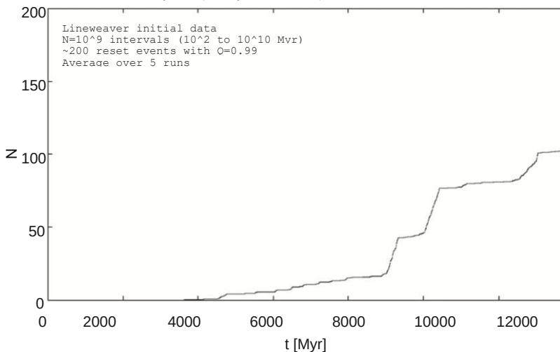
Рисунок 18.1 Пример глобальных механизмов сброса, вызывающих фазовый переход в очень упрощенной модели Млечного Пути, первоначально опубликованный в работе Вукотича и Цирковича (2007). Множеству участков присваивается временной масштаб для возникновения разумной цивилизации (выбранный равномерно в диапазоне от 10^8 до 10^{16} лет). При наличии соответствующего распределения возрастов и вероятности Q того, что событие перезагрузки уничтожит шансы данного участка на развитие цивилизации, можно вызвать фазовый переход
