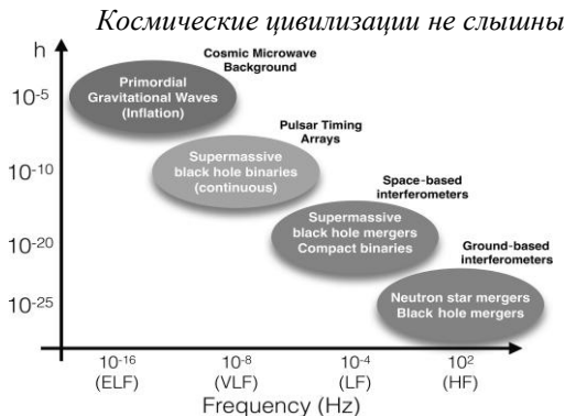
Рисунок 21.4 Схема астрофизических источников гравитационных волн в зависимости от частоты и деформации волн.
