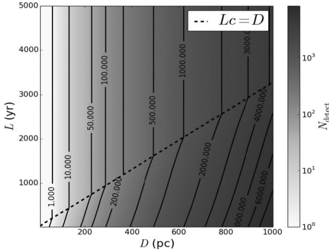
Рисунок 27.2 Количество обнаруживаемых цивилизаций как функция времени жизни трансляции цивилизации L и дальности трансляции D (см. уравнение (27.6)). Заметим, что для долгоживущих сигналов обнаруживаемость зависит только от дальности. Как только Lc \leq D (пунктирная линия), обнаруживаемость зависит от ширины сферической оболочки, создаваемой изотропным сигналом.
