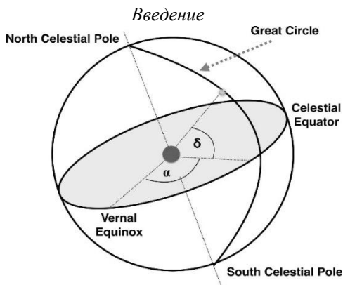
Рисунок 2.1 Экваториальная система координат. Небесная сфера определяется небесным экватором (плоскостью, содержащей экватор Земли), небесными северным и южным полюсами, перпендикулярными этой плоскости, и контрольным местоположением на экваторе (точка весеннего равноденствия). Затем с помощью этой системы можно рассчитать прямое восхождение \alpha и склонение \delta с соответствующим расчетом часового угла, который учитывает вращение Земли.
