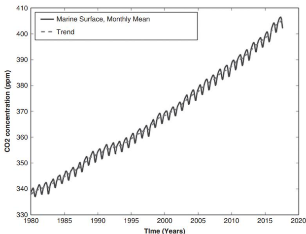
Рисунок 13.1 Уровни \text{CO}_2 (в частях на миллион), измеренные на нескольких участках морской поверхности и подвергнутые скользящему среднему (с использованием семи смежных точек). Источник данных: Ed Dlugokencky and Pieter Tans, NOAA/ESRL ( www.esrl.noaa.gov/gmd/ccgg/trends/ )
