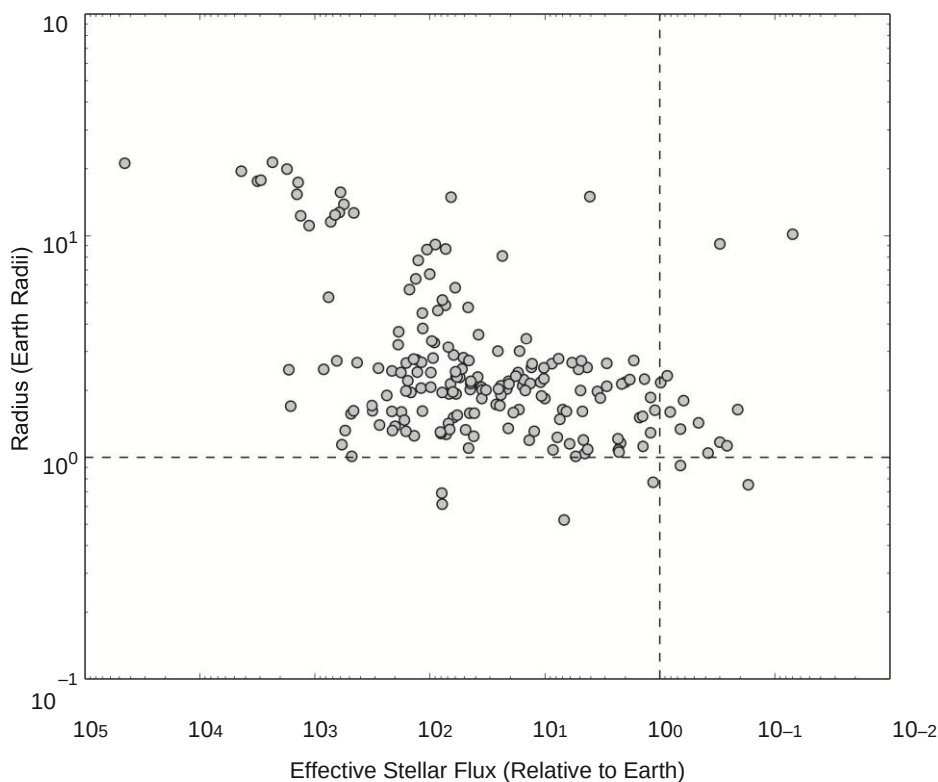
Рисунок 4.9 Радиус экзопланеты (в радиусах Земли) в зависимости от эффективного потока звездного излучения, где I = поток звездного излучения, принимаемый Землей. Пунктирные линии показывают значения для Земли. Данные предоставлены Архивом экзопланет НАСА.
