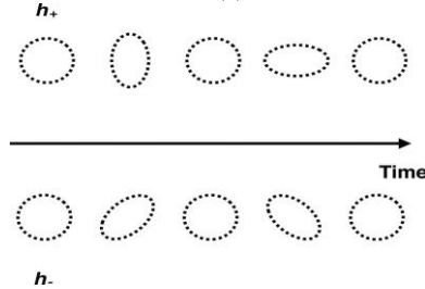
Рисунок 21.2 Два состояния поляризации гравитационных волн. Круговое кольцо из масс деформируется при прохождении гравитационной волны с (вверху) возмущением h^+ и (внизу) h^- возмущением.
