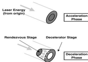
Рисунок 19.5 Схема концепции Форварда (Forward, 1984) с двумя парусами для фаз ускорения и замедления. Лазерный свет от источника света (Солнце, толстые стрелки) воздействует на оба паруса конструктивно во время фазы ускорения и деструктивно во время замедления, при этом результирующая передача импульса на парус сближения происходит за счет фотонов, отклоненных парусом замедления.
