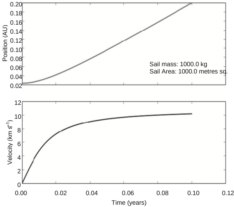
Рисунок 19.4 Изменение положения и скорости солнечного паруса массой 1 тонна (площадь 1000 \text{m}^2 ) по мере его ускорения при удалении от Солнца, начиная с расстояния в 5 солнечных радиусов.
