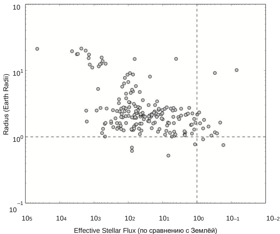
Рисунок 4.9 Радиус экзопланеты (в радиусах Земли) в зависимости от эффективного потока звёздного излучения, где I = поток звёздного излучения, принимаемый Землей. Пунктирные линии показывают значения для Земли. Данные предоставлены Архивом экзопланет НАСА.
