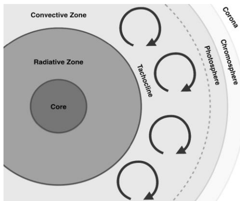
Рисунок 10.1 Внутреннее строение Солнца. Внутри ядра водород превращается в гелий в результате термоядерного синтеза. Две основные зоны звёздной атмосферы — радиационная и конвективная — соединены в тахоклине. Фотоны, достигнув фотосферы, свободно вырываются из атмосферы, проходя через горячую хромосферу и за пределы корональной плазмы.
