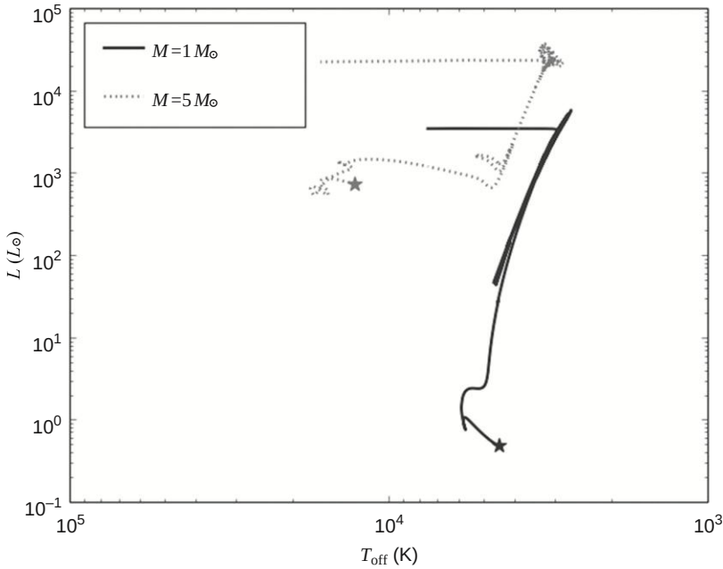
Рисунок 10.3 Эволюция звезды массой 1 M_{\odot} (сплошная линия) и звезды массой 5 M_{\odot} (пунктирная линия) на диаграмме Герцшпрунга. Мы начинаем движение с обеих звёзд на главной последовательности (через ветвь субгигантов к ветви красных гигантов (RGB)). Звезда массой 1 M_{\odot} эволюционирует вдоль главной последовательности и, начиная с главной последовательности, начинает термоядерный синтез гелия в своем ядре, затем опускается вниз и присоединяется к асимптотической ветви гигантов (AGB), которая точно следует за RGB. Достигнув вершины AGB (когда горение гелия в ядре прекращается), звезда эволюционирует в сторону фазы планетарной туманности/белого карлика (не показано на графике). Звезда массой 5 M_{\odot} быстро перескакивает через «синюю петлю», прежде чем присоединиться к AGB, поскольку она способна начать термоядерный синтез гелия в углерод еще до того, как покинет RGB. Данные получены в рамках проекта MESA Isochrones and Stellar Tracks с использованием кода MESA для моделирования эволюции звёзд.
