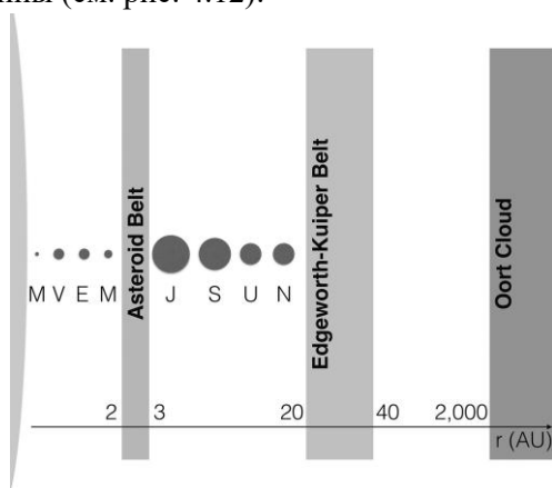
Рисунок 4.12 Положения основных семейств астероидов и комет в Солнечной системе относительно восьми известных планет..
