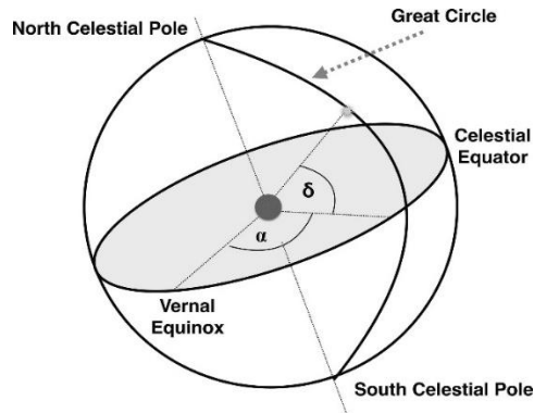
Рисунок 2.1 Экваториальная система координат. Небесная сфера определяется небесным экватором (плоскостью, содержащей экватор Земли), небесными северным и южным полюсами, перпендикулярными этой плоскости, и контрольным местоположением на экваторе (точка весеннего равноденствия). Затем с помощью этой системы можно рассчитать прямое восхождение \alpha и склонение \delta с соответствующим расчетом часового угла, который учитывает вращение Земли.
