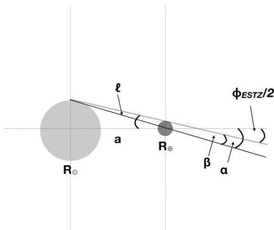
Рисунок 27.1 Транзитная зона Земли, определяемая как угловая область \phi_{ESTZ} = 2(\alpha - \beta) \sim R/a в пределах R \gg R_{\oplus} .
