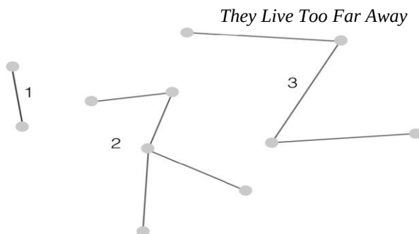
Рисунок 22.2 Пример графа с тремя связными компонентами.
