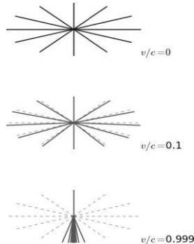
Рисунок 19.7 Иллюстрация релятивистской абберации. Свет излучается источниками, находящимися в состоянии покоя, вдоль радиальных линий зрения в направлении нашего космического аппарата, также находящегося в состоянии покоя (верхний рисунок). Источники, расположенные немного позади этих точек, будут по-прежнему видны наблюдателю, движущемуся на космическом аппарате со скоростью 0,1c (средний рисунок). При высоких релятивистских скоростях поле зрения наблюдателя приближается к 360^\circ (нижний рисунок).
