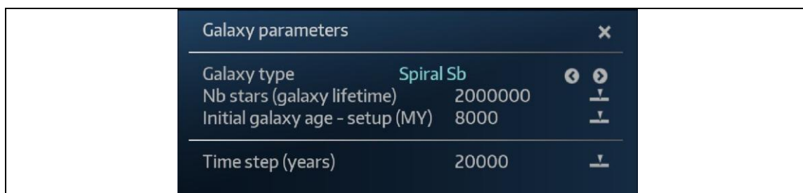
Рисунок 42. Параметры галактик
