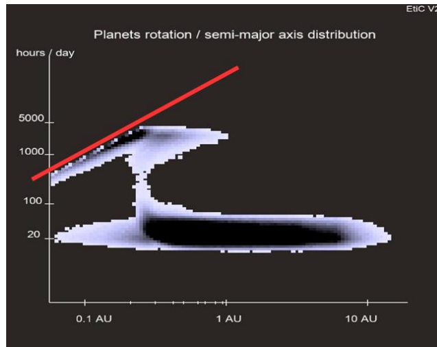
Рисунок 20. Вращение планеты как функция semi-major axis
