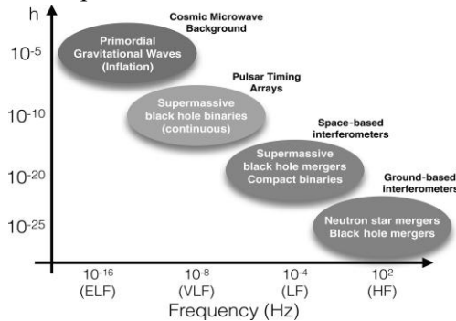
Рисунок 21.4 Схема астрофизических источников гравитационных волн в зависимости от частоты и деформации волны.
