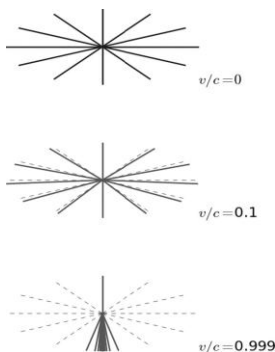
Рисунок 19.7 Иллюстрация релятивистской аберрации. Свет излучается источниками, находящимися в состоянии покоя, вдоль радиальных линий зрения в направлении нашего космического аппарата, также находящегося в состоянии покоя (верхний рисунок). Источники, расположенные немного позади этих точек, будут по-прежнему видны наблюдателю, движущемуся на космическом аппарате со скоростью 0,1c (средний рисунок). При высоких релятивистских скоростях поле зрения наблюдателя приближается к 360^\circ (нижний рисунок).
