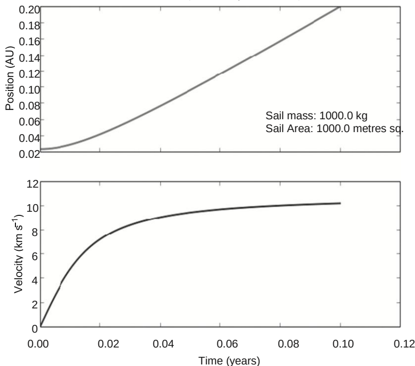
Рисунок 19.4 Изменение положения и скорости солнечного паруса массой 1 тонна (площадь 1000 \text{ м}^2 ) по мере его ускорения при удалении от Солнца, начиная с расстояния в 5 солнечных радиусов.
