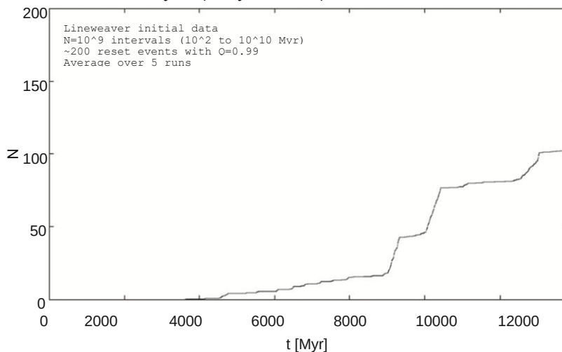
Рисунок 18.1 Пример глобальных механизмов регулирования, вызывающих фазовый переход в очень упрощенной модели Млечного Пути, первоначально опубликованный в работе Вукотича и Цирковича (2007). Множеству участков присваивается временной масштаб для возникновения разумной цивилизации (выбранный равномерно в диапазоне от 10^8 до 10^{16} лет). При наличии соответствующего распределения возрастов и вероятности Q того, что событие перезагрузки уничтожит шансы данного участка на развитие цивилизации, можно вызвать фазовый переход в количестве разумных цивилизаций N . Количество участков с разумной цивилизацией подавляется на ранних этапах из-за высокой частоты событий перезагрузки. По мере уменьшения частоты событий перезагрузки в этой простой модели в конечном итоге может появиться больше цивилизаций.
