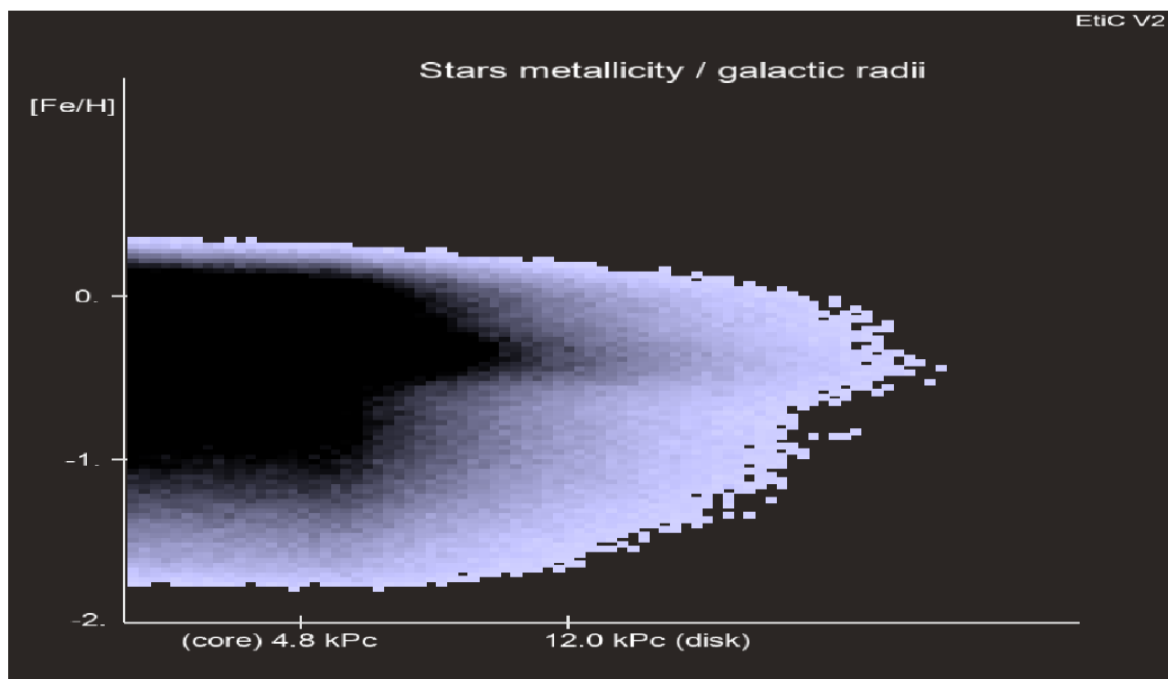
Рис. 13 – Металличность звёзд как функция галактического радиуса
