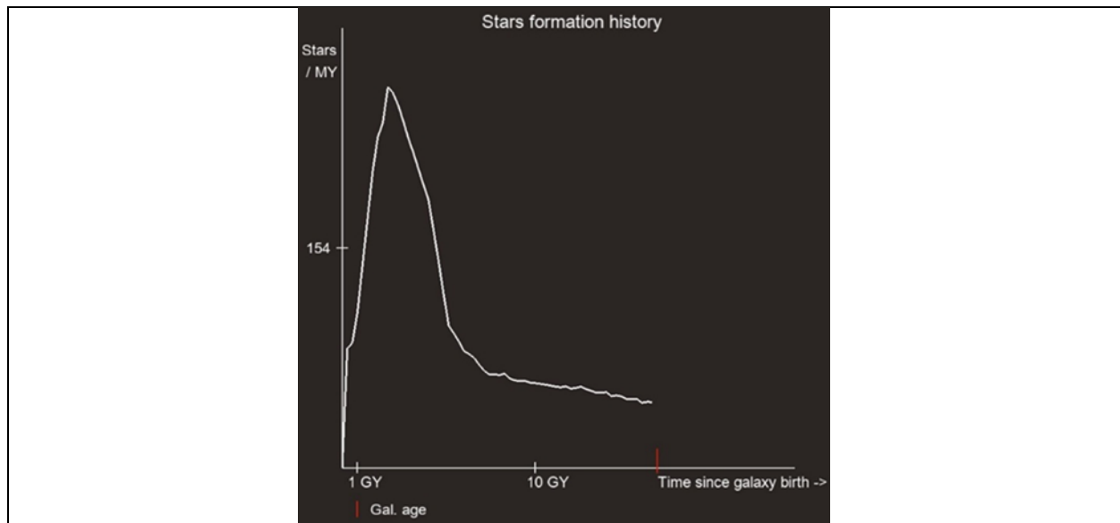
Рисунок 9. История звёздообразования
