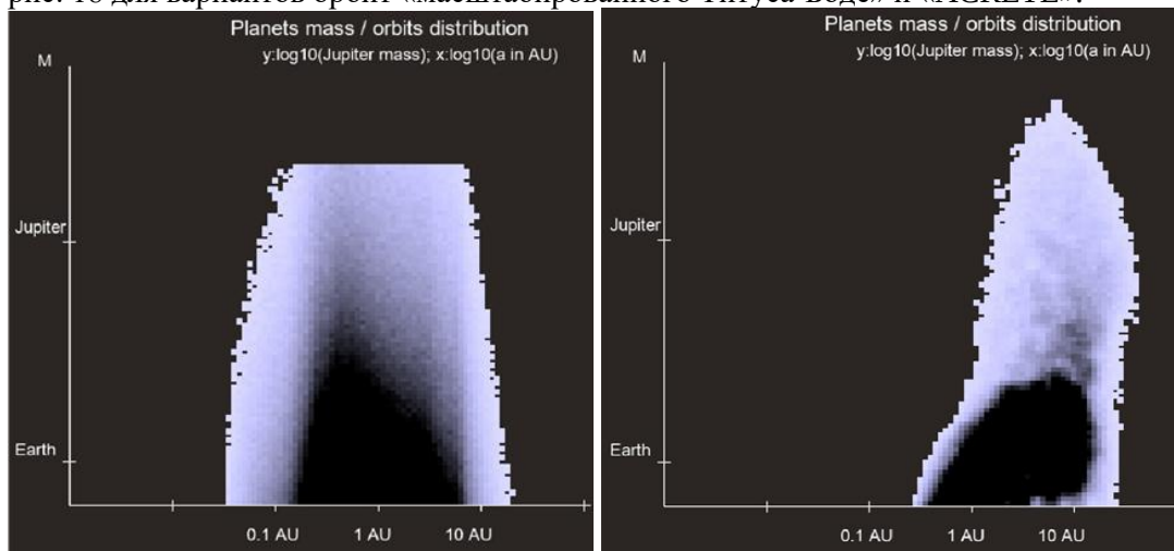
Рисунок 18. Распределение планет по большим полуосям справа: вариант "Акрет", ниже: "масштабированная модель Титуса-Бодя"
