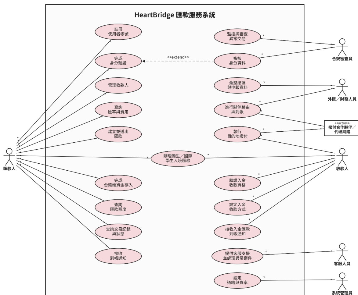
(圖 1 心橋匯款服務系統之角色與使用案例關係圖)
