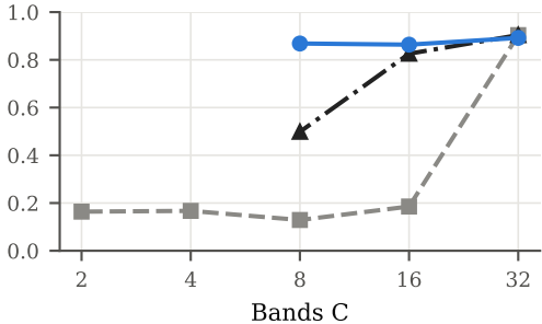
(b) Macro-F1
