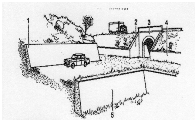
FOTO 48 – Murature esterne: 1. m. di controripa; 2. m. d'ala. 3. m. di testa, 4. m. di risolto; 5. m. di scarpa.
