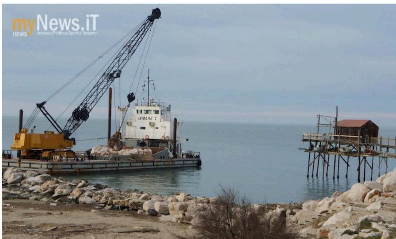
Macchine che eseguono il lavoro di Dragaggio
