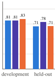
micro-F1
