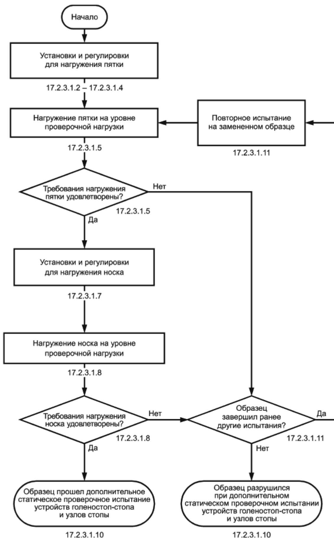
Рисунок 19 - Блок-схема дополнительного статического проверочного испытания голеностопных узлов
