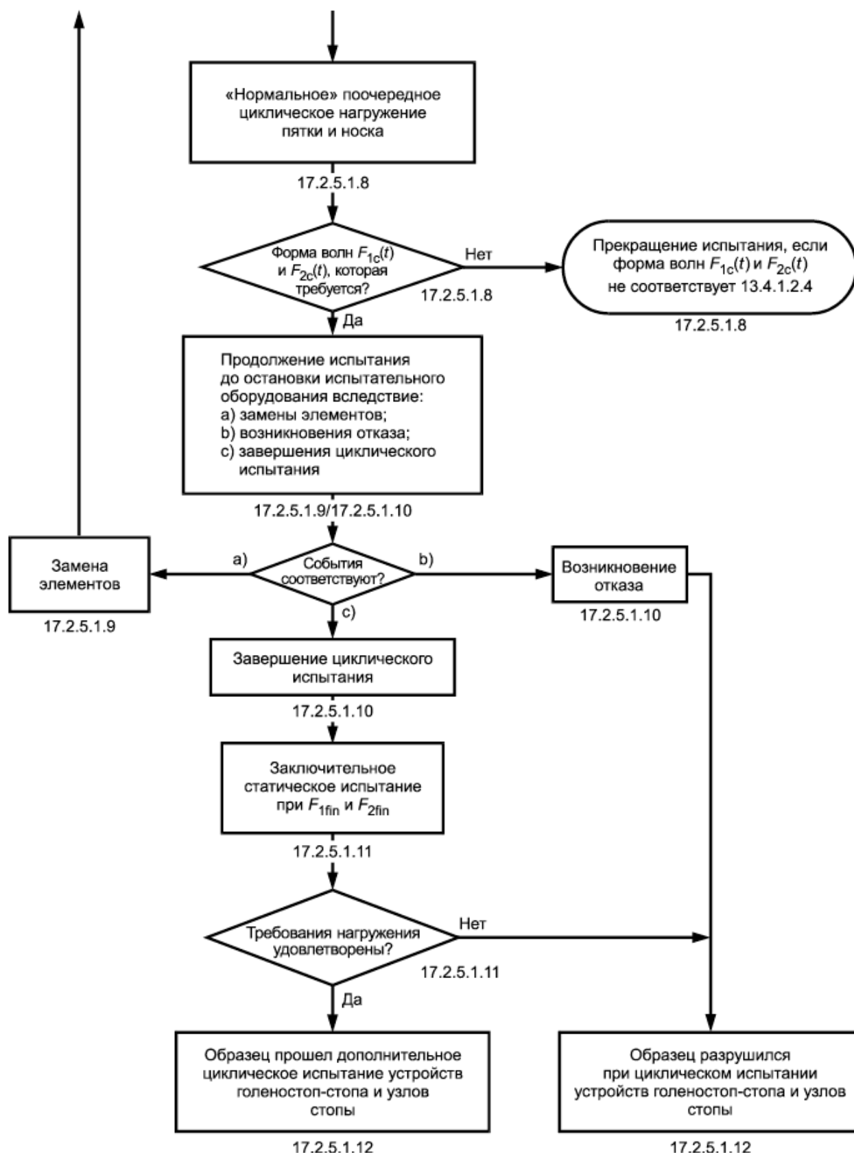
Рисунок 22 - Блок-схема дополнительного циклического испытания голеностопных узлов и узлов стоп, установленного в 17.2.5.1. Продолжение рисунка 21
