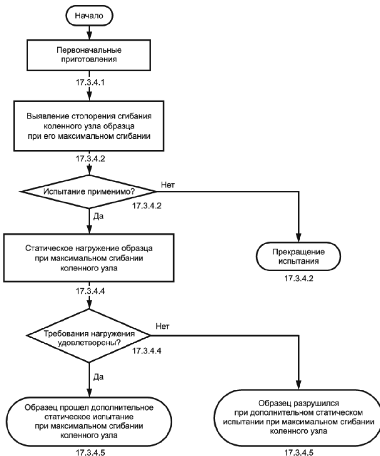
Рисунок 23 - Блок-схема дополнительного статического испытания на предельную прочность при максимальном сгибании коленных узлов и смежных с ними элементов, установленного в 17.3.4 - крепления этих сборок к проксимальной и к дистальной частям протезов и установки коленного узла в протезе;
