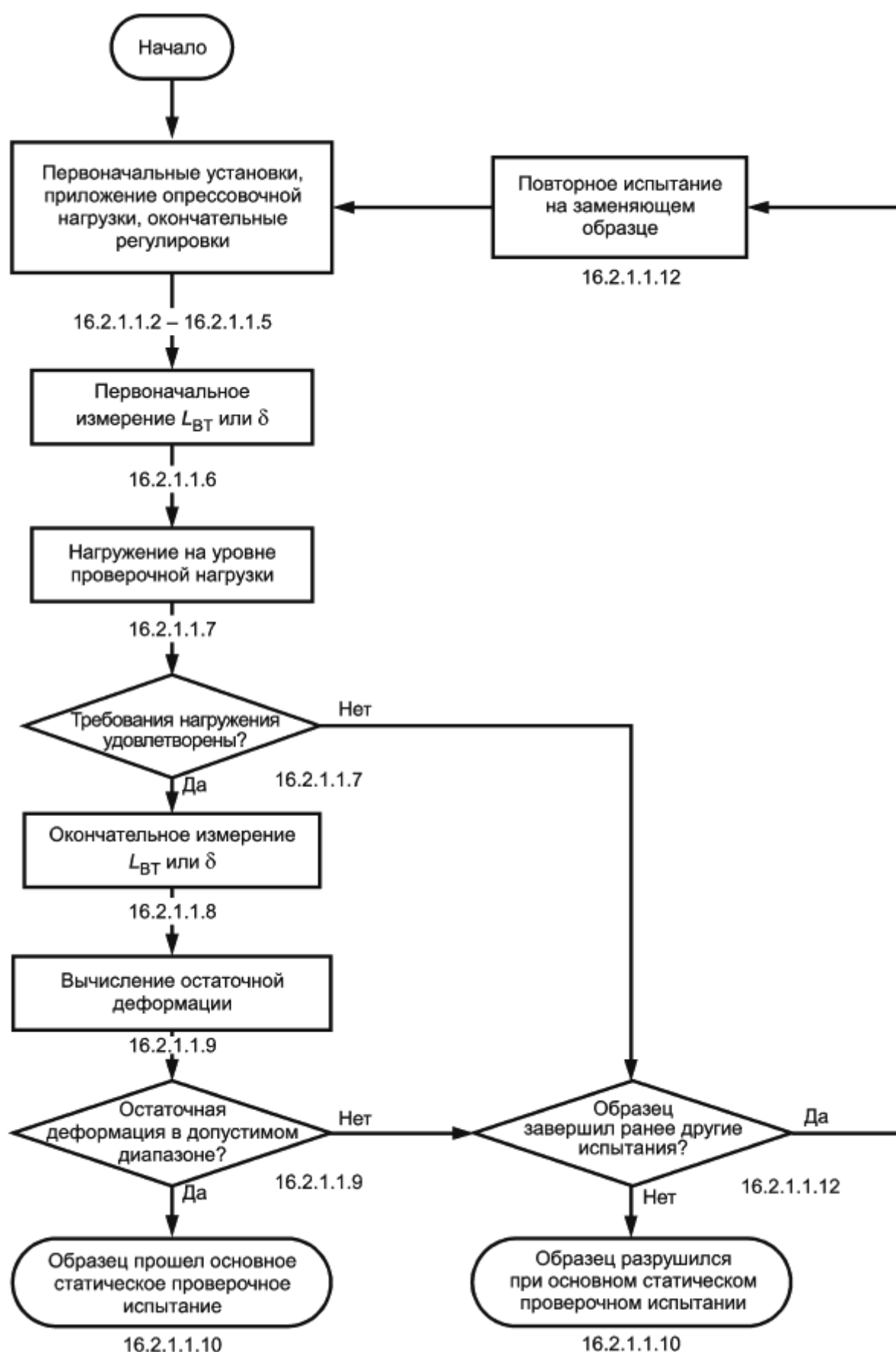
Рисунок 13 - Блок-схема основного статического проверочного испытания, установленного в 16.2.1.1 16.2.1.1.2 Подготавливают и центрируют образец из группы, указанный для данного испытания в
