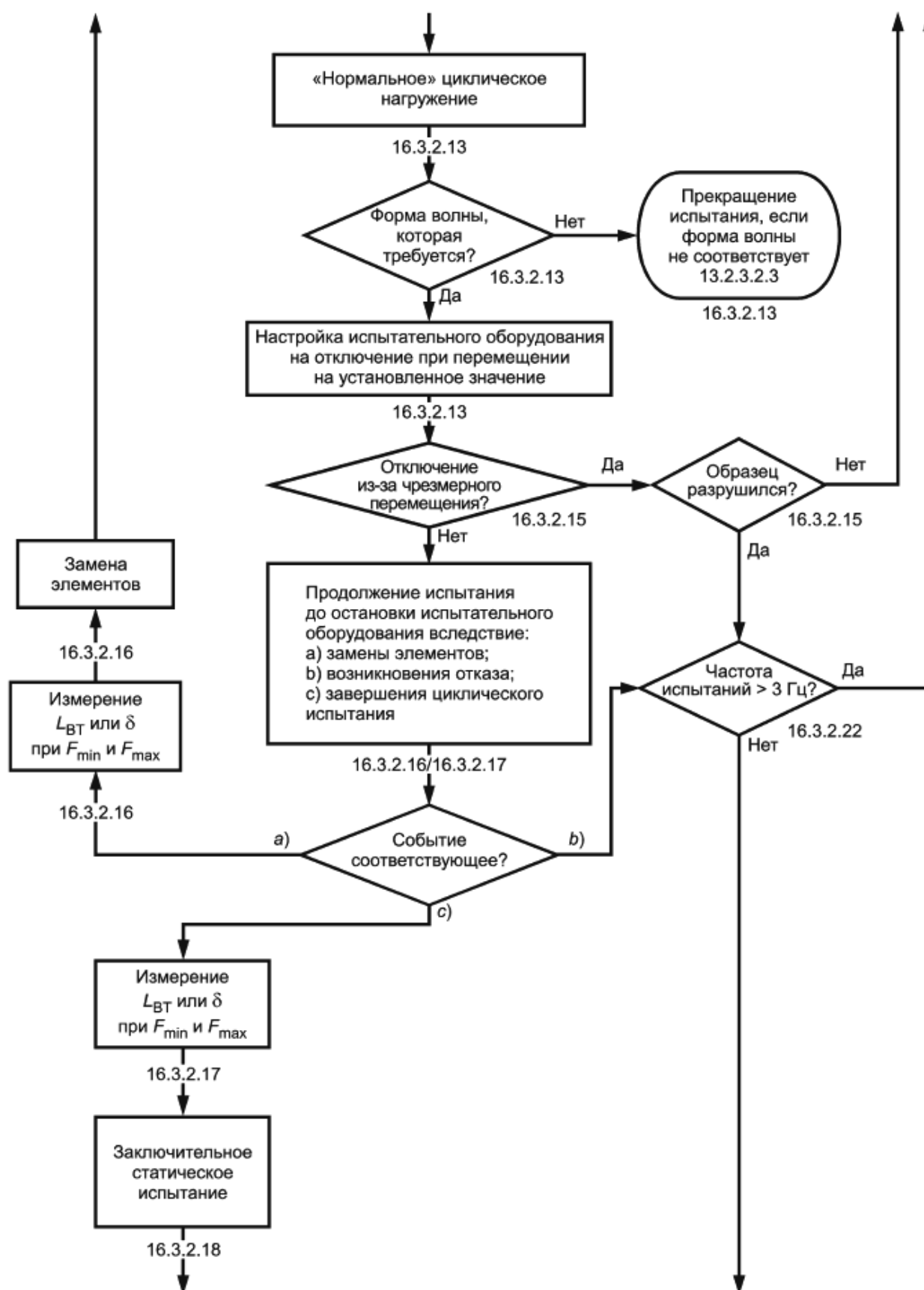
Рисунок 16 - Блок-схема основного циклического испытания, установленного в 16.3.2. Продолжение рисунка 15 и продолжение на рисунке 17
