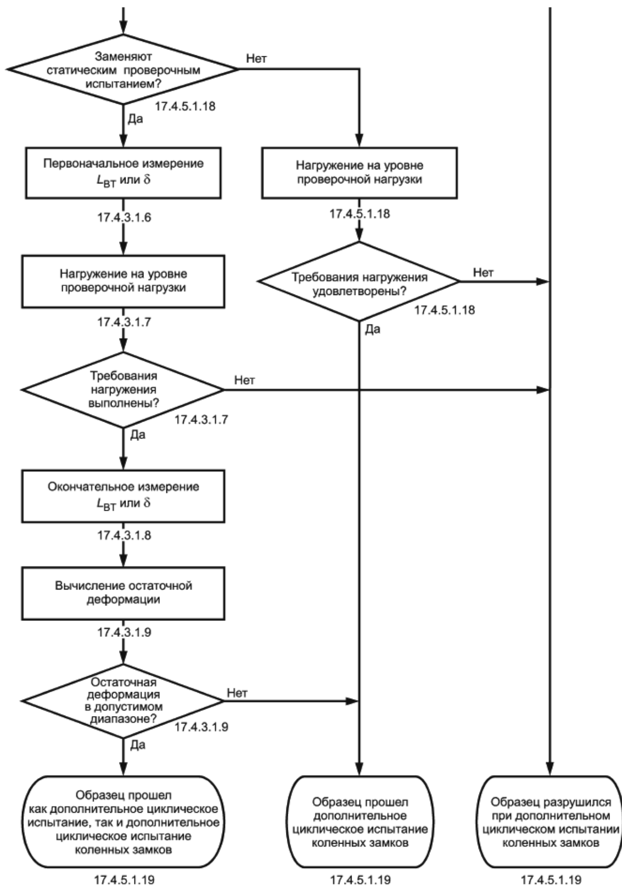
Рисунок 28 - Блок-схема дополнительного циклического испытания замков коленных узлов,
