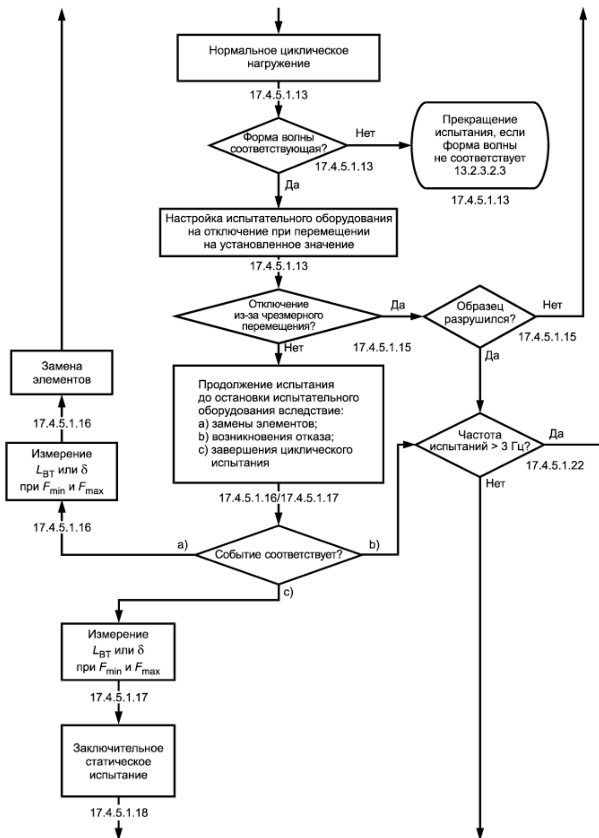
Рисунок 27 - Блок-схема дополнительного циклического испытания замков коленных узлов, установленного в 17.4.5.1
