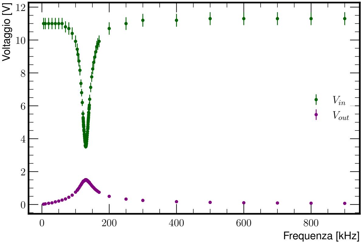
Tensioni misurate V_{in} e V_{out}
