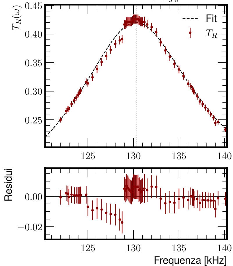
Zoom vicino a f_0
