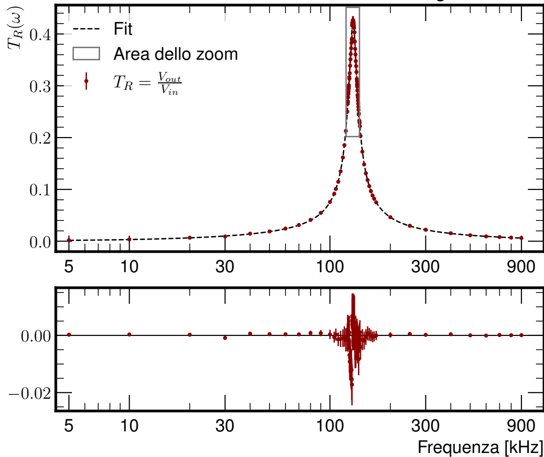
Fit funzione di trasferimento con asse logaritmico
