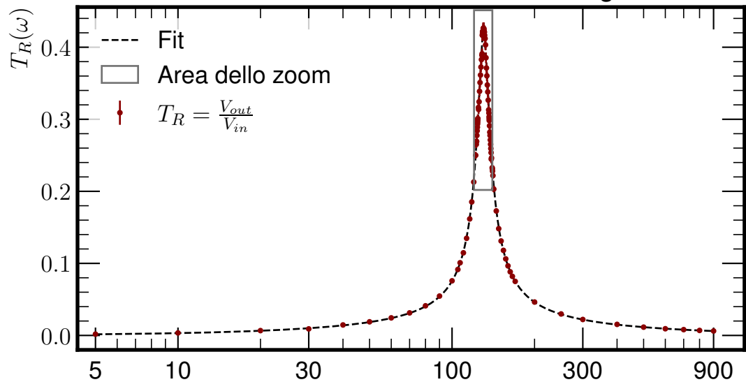
Fit funzione di trasferimento con asse logaritmico
