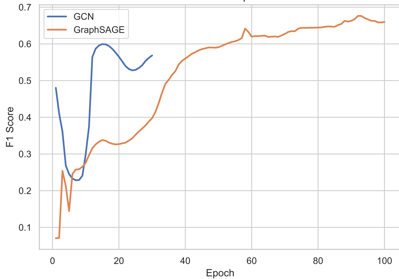
F1 Score over Epochs
