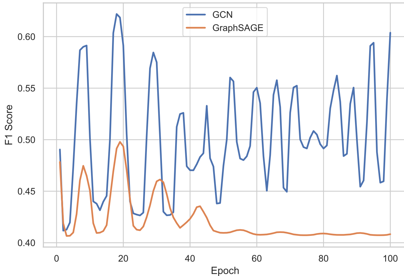
F1 Score over Epochs
