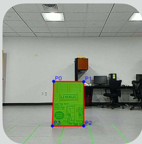
Edge Detection (OWL ViT + SAM)
