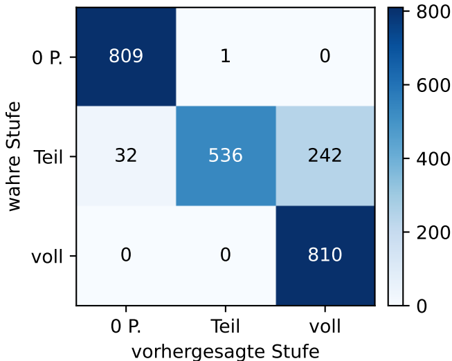
Konfusionsmatrix
