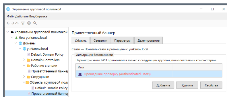
Рисунок 54 — Фильтрация безопасности объекта GPO
