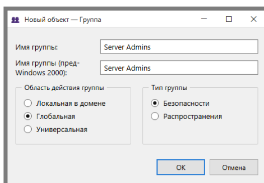
Рисунок 57 — Создание доменной группы безопасности
