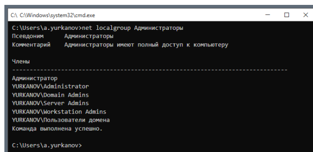
Рисунок 59 — Состав локальной группы администраторов на клиенте
