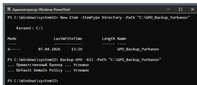
Рисунок 55 — Резервное копирование объектов GPO
