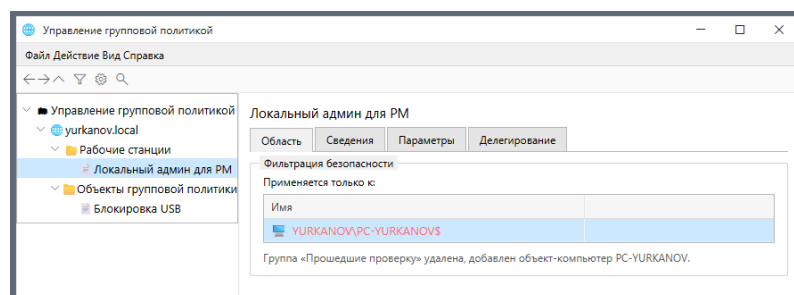
Рисунок 64 — Фильтрация политики на конкретный компьютер
