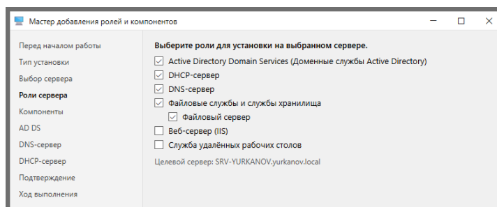
Рисунок 24 — Выбор ролей: AD DS, DNS, DHCP и файловый сервер
