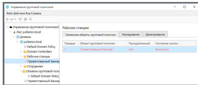
Рисунок 50 — Привязка GPO к подразделению
