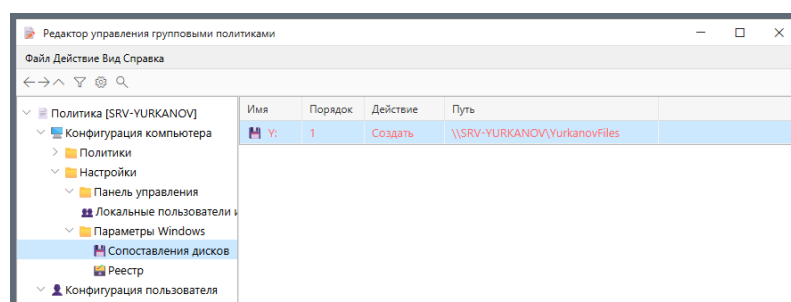
Рисунок 60 — Сопоставление сетевого диска Y: групповой политикой
