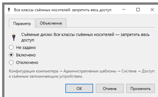
Рисунок 65 — Включение запрета доступа к съёмным носителям
