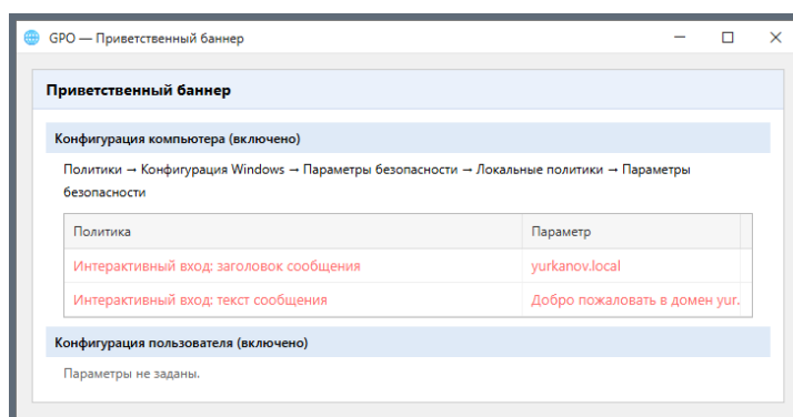
Рисунок 53 — Отчёт по настройкам GPO
