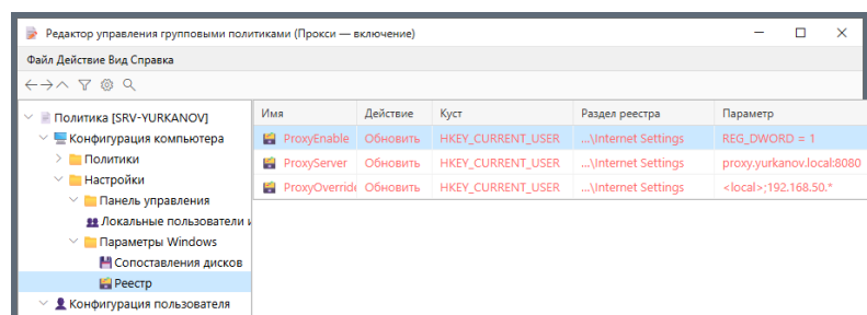
Рисунок 62 — Включение прокси-сервера через реестр GPO
