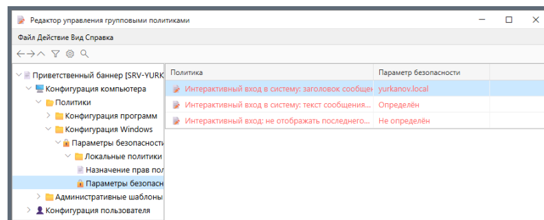
Рисунок 48 — Путь к параметрам баннера в редакторе GPO
