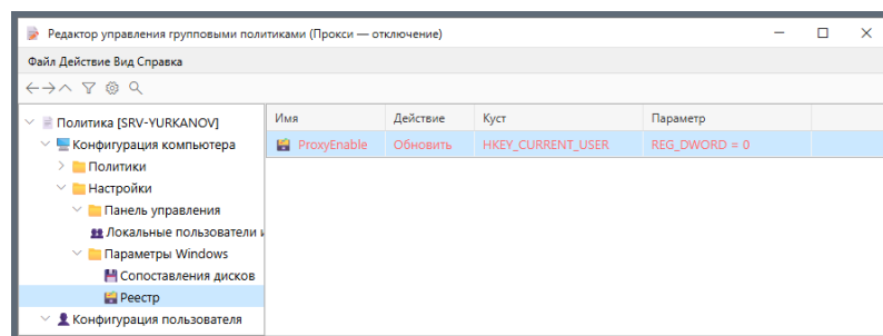
Рисунок 63 — Отключение прокси-сервера
