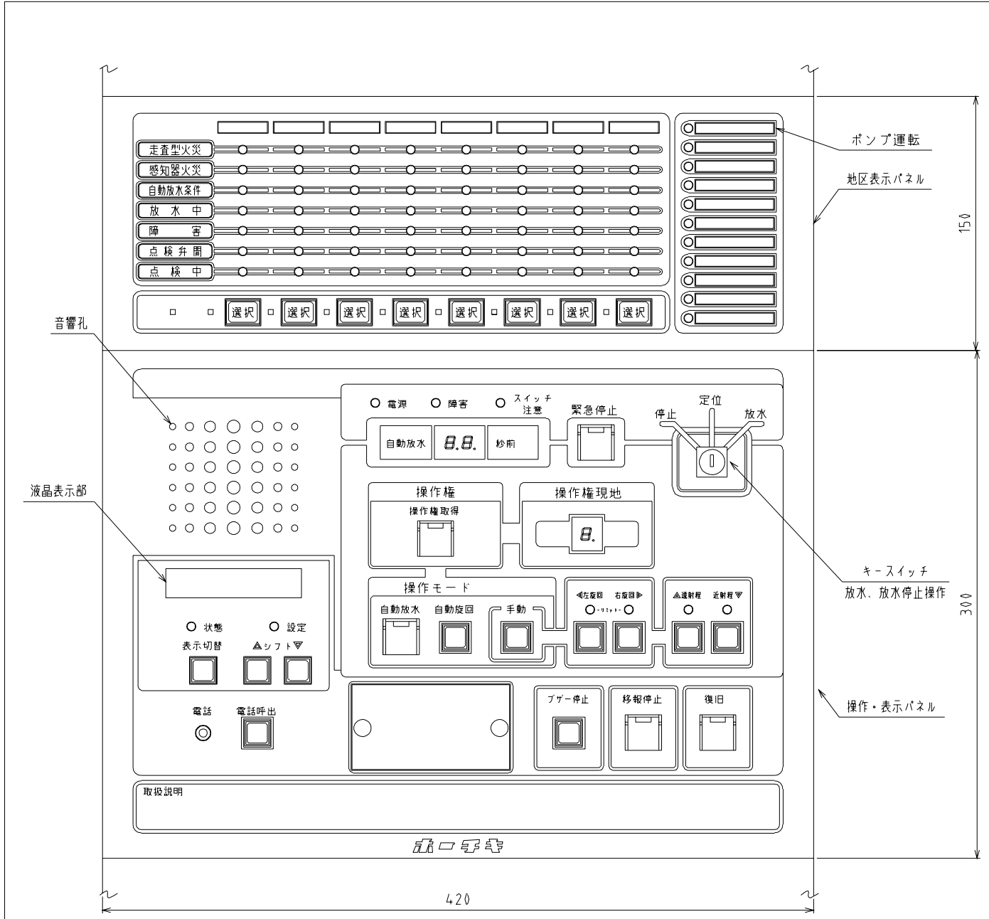
本図は、GDB-AAW8の地区表示パネル、操作・表示パネルの内容を示した図面です。
